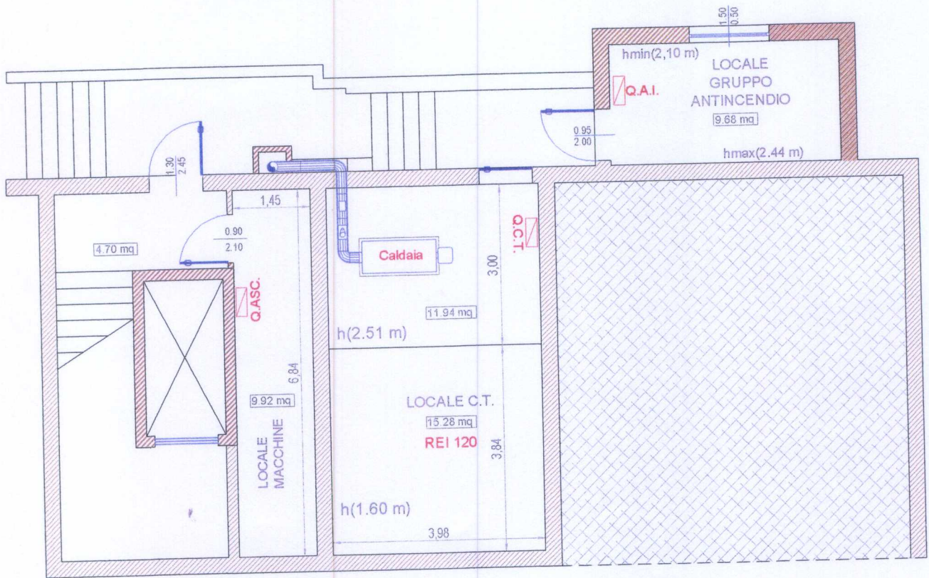
PLANIMETRIA LOCALE SEMINTERRATO scala 1:100
