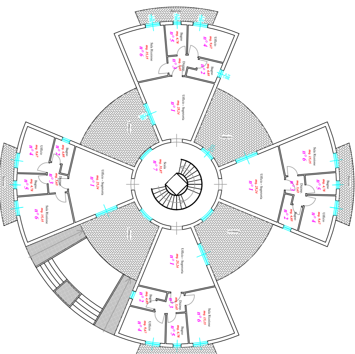
STATO DI PROGETTO FABBRICATO "A" - Piano Primo Riferito & Primo - NON RESIDENZIALE
