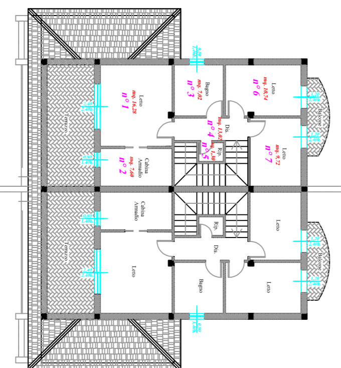
STATO DI PROGETTO FABBRICATO Bimembre PIANTA PIANO RALZATO
