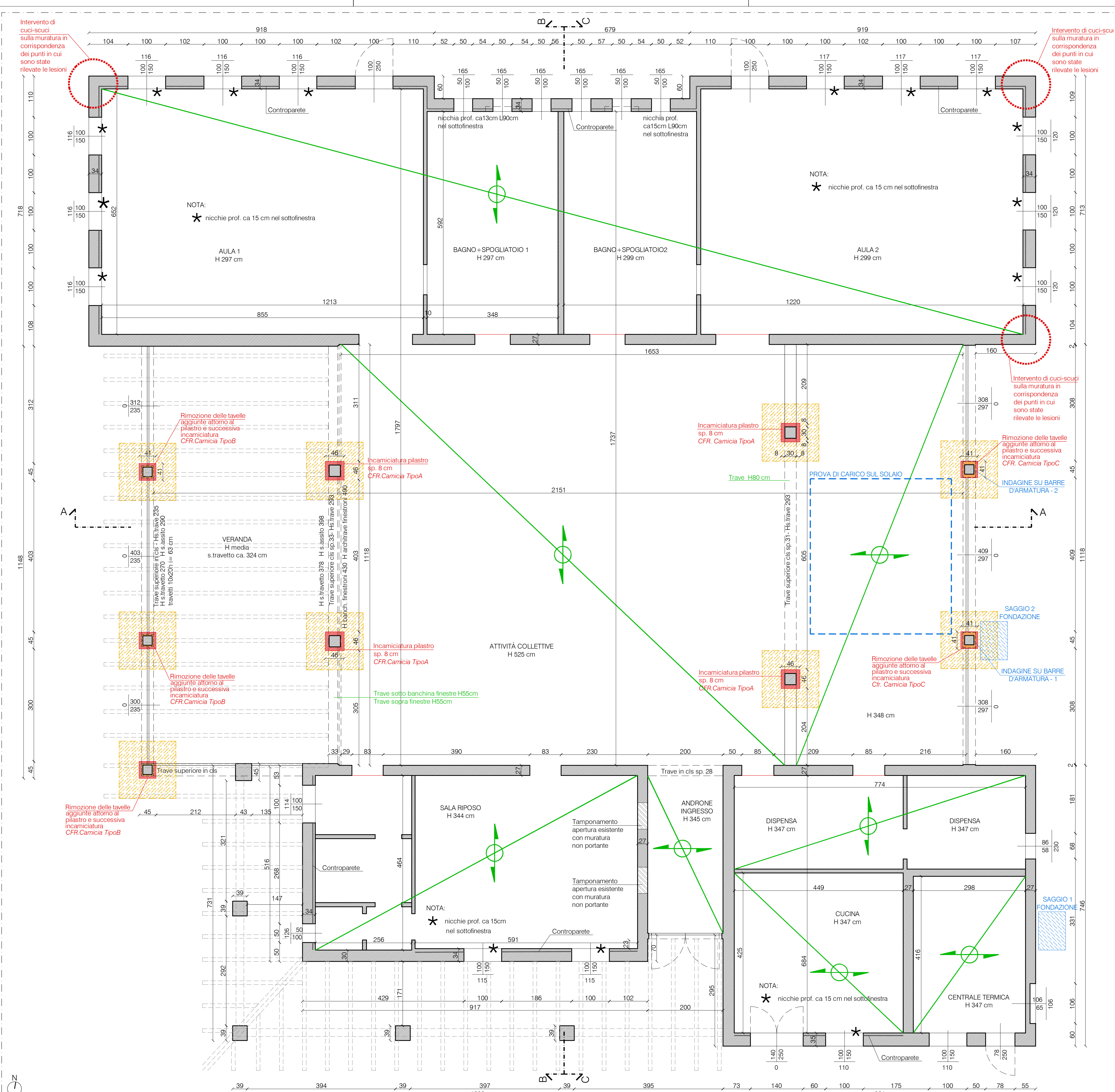
STATO DI PROGETTO - PIANTE PIANO TERRA CON NOTAZIONI INERENTI LE STRUTTURE (IN VERDE), LOCALIZZAZIONE DI ALCUNE PROVE ESEGUITE SU DI ESSE (IN BLU) E IDENTIFICAZIONE DEGLI INTERVENTI FUNZIONALI ALL'IDONEITÀ STATICA (EVIDENZIATI IN ROSSO) : SCALA 1:50
