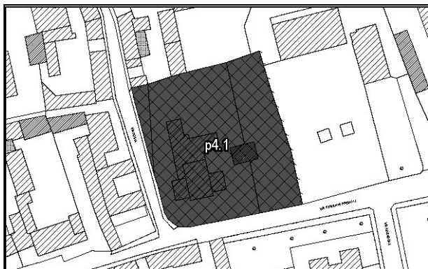
Figura 7 Scuola materna. Planimetria
