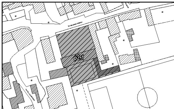
Figura 71 Oratorio. Planimetria
