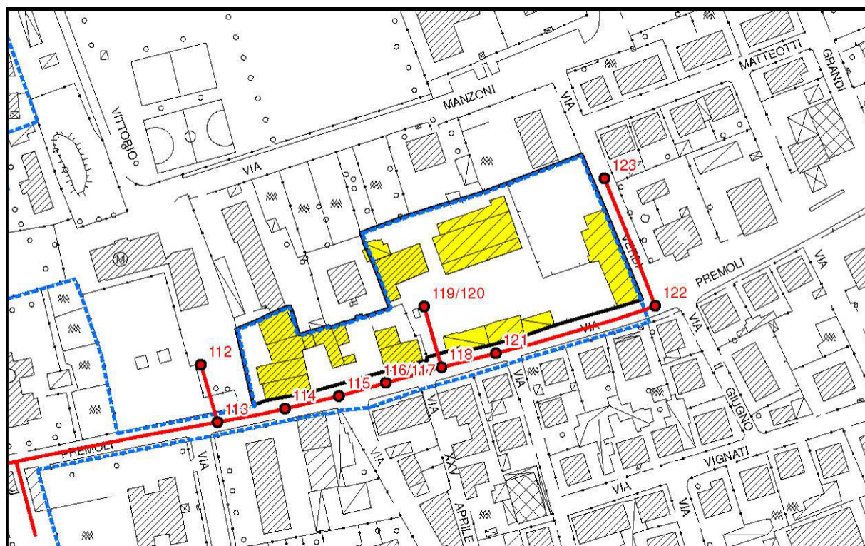
Figura 17 Isolato 7 (Via G. Premoli, Via Verdi): planimetria con punti di ripresa fotografici
