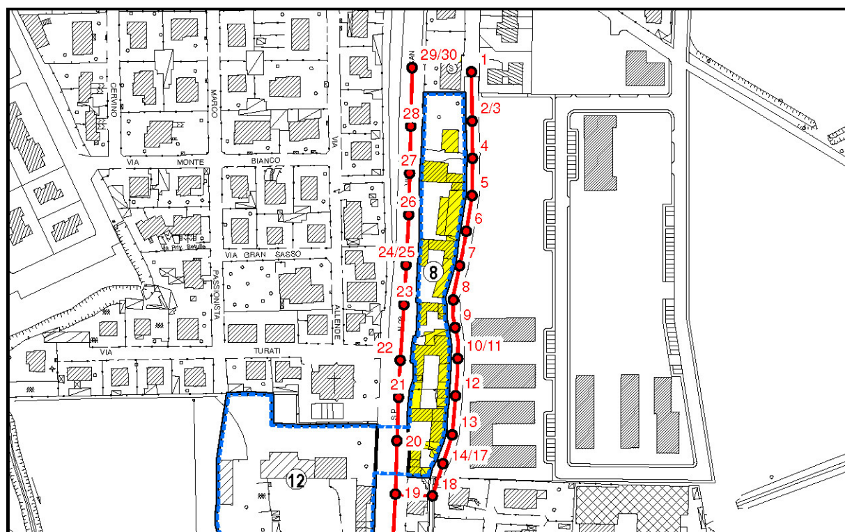
Figura 19 Isolato 8 (Motta Vigana, SP 23): planimetria con punti di ripresa fotografici
