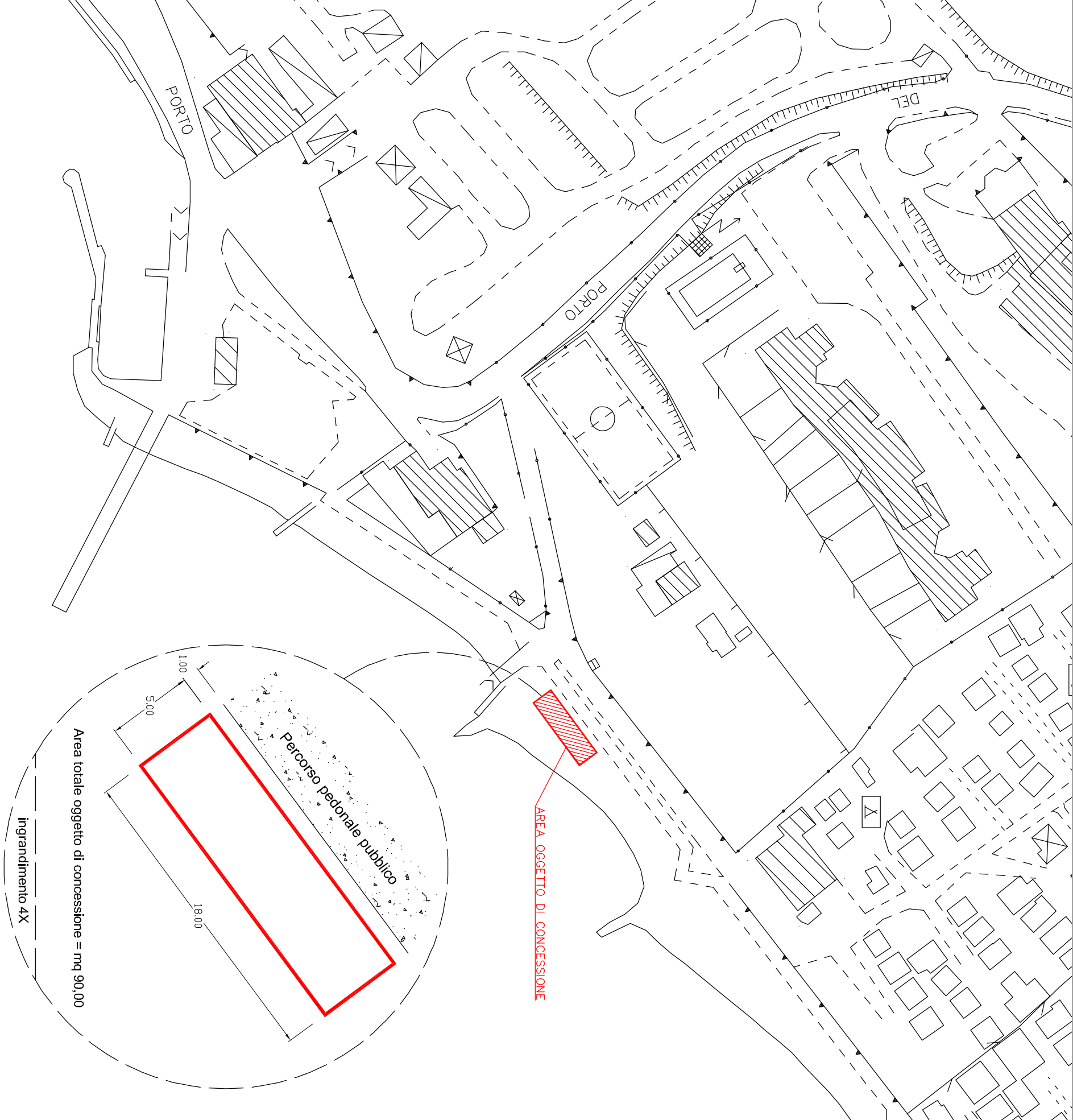
TAVOLA N. 1 (rif. B24) SCHEMA PLANIMETRICO AREA IN CONCESSIONE Comune di Moniga d/G (scala 1:1000)
