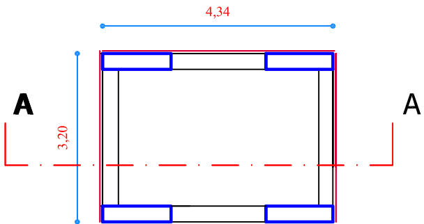
PIANTE COPERTURA
