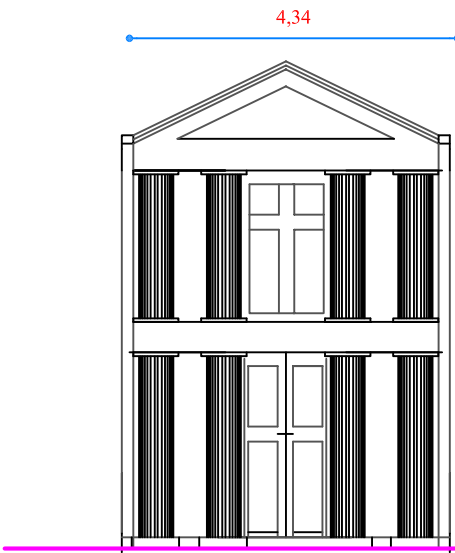
PROSPETTO
