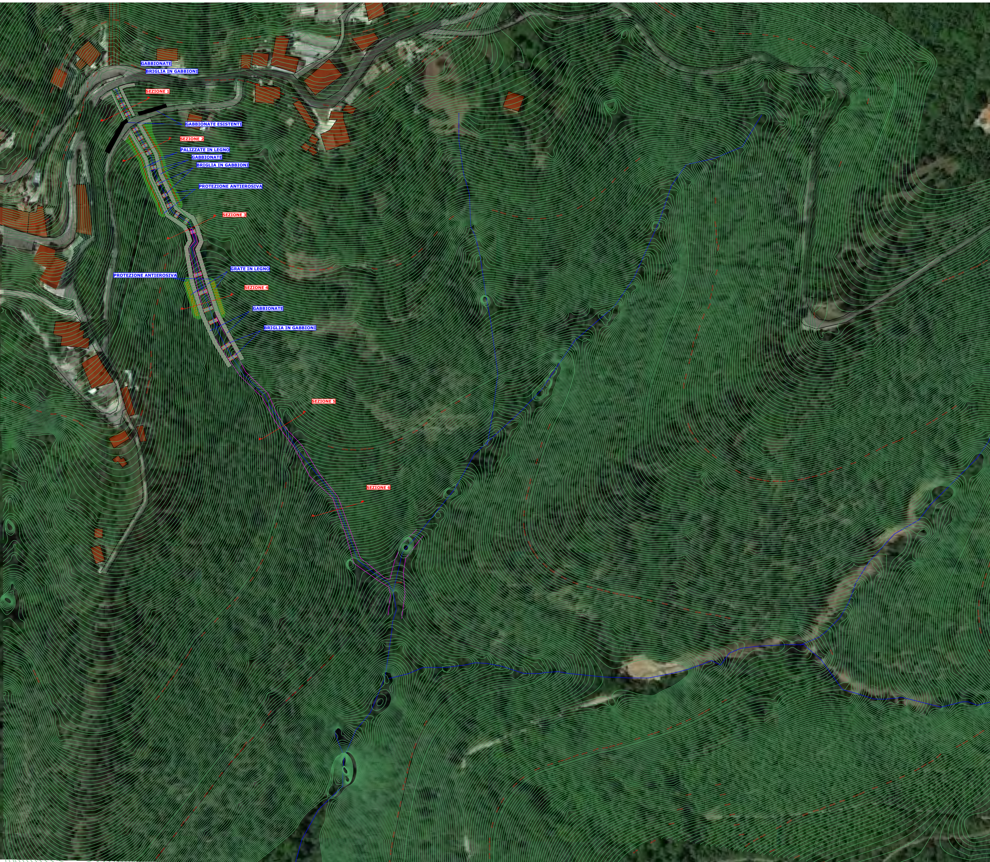
OROFOTO DELL'AREA CON UBICAZIONE INTERVENTI DI PROGETTO - Scala 1:2'000
