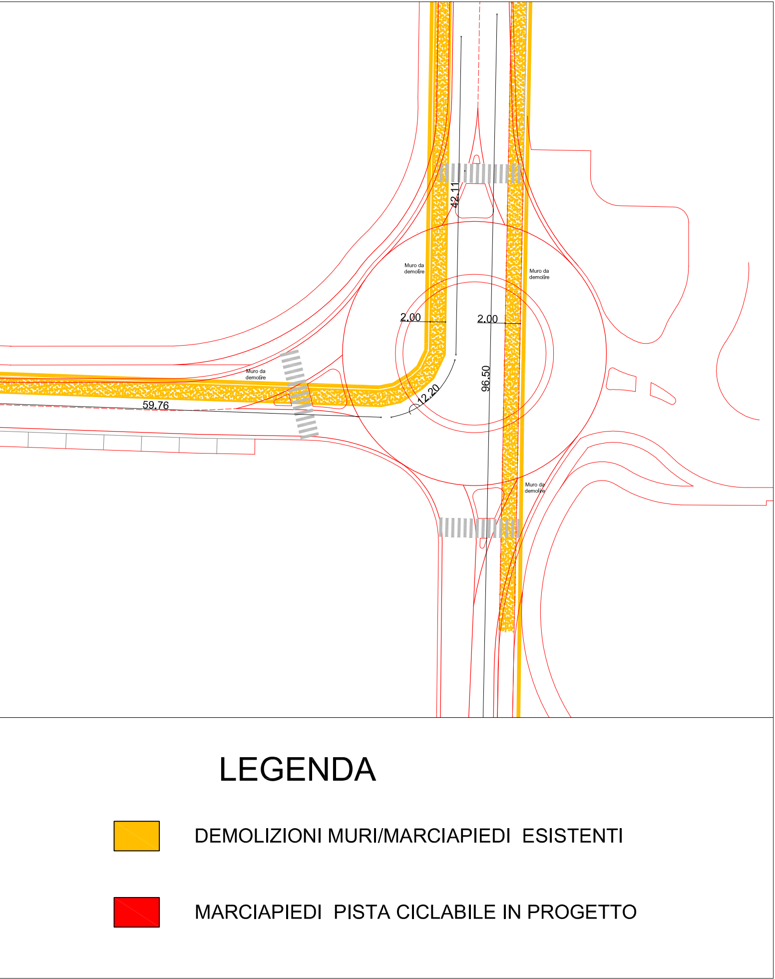
PIANTA ROTATORIA SUD scala 1:500 sovrapposizione nuovi interventi/demolizioni
