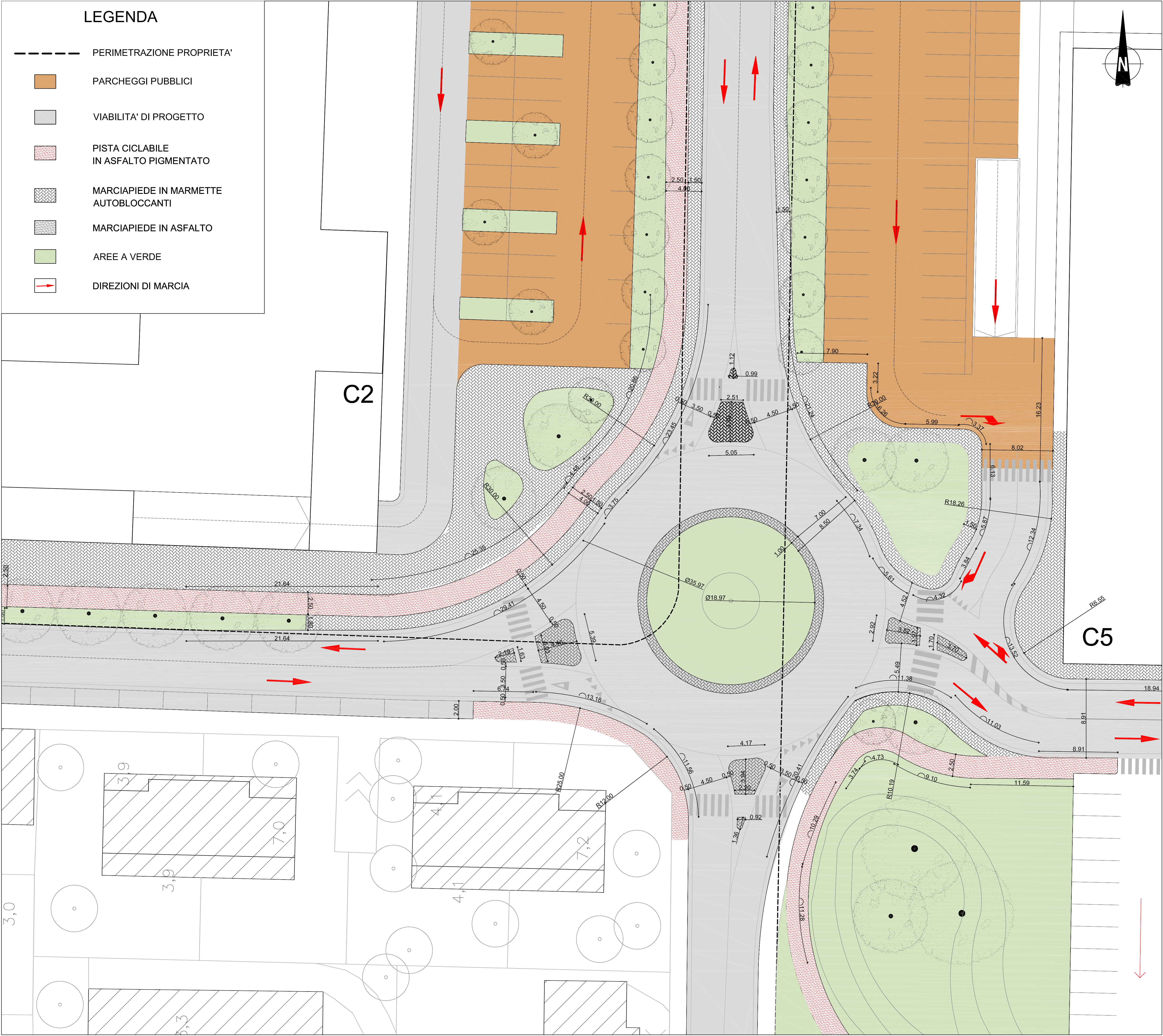
PIANTA ROTATORIA SUD scala 1:200
