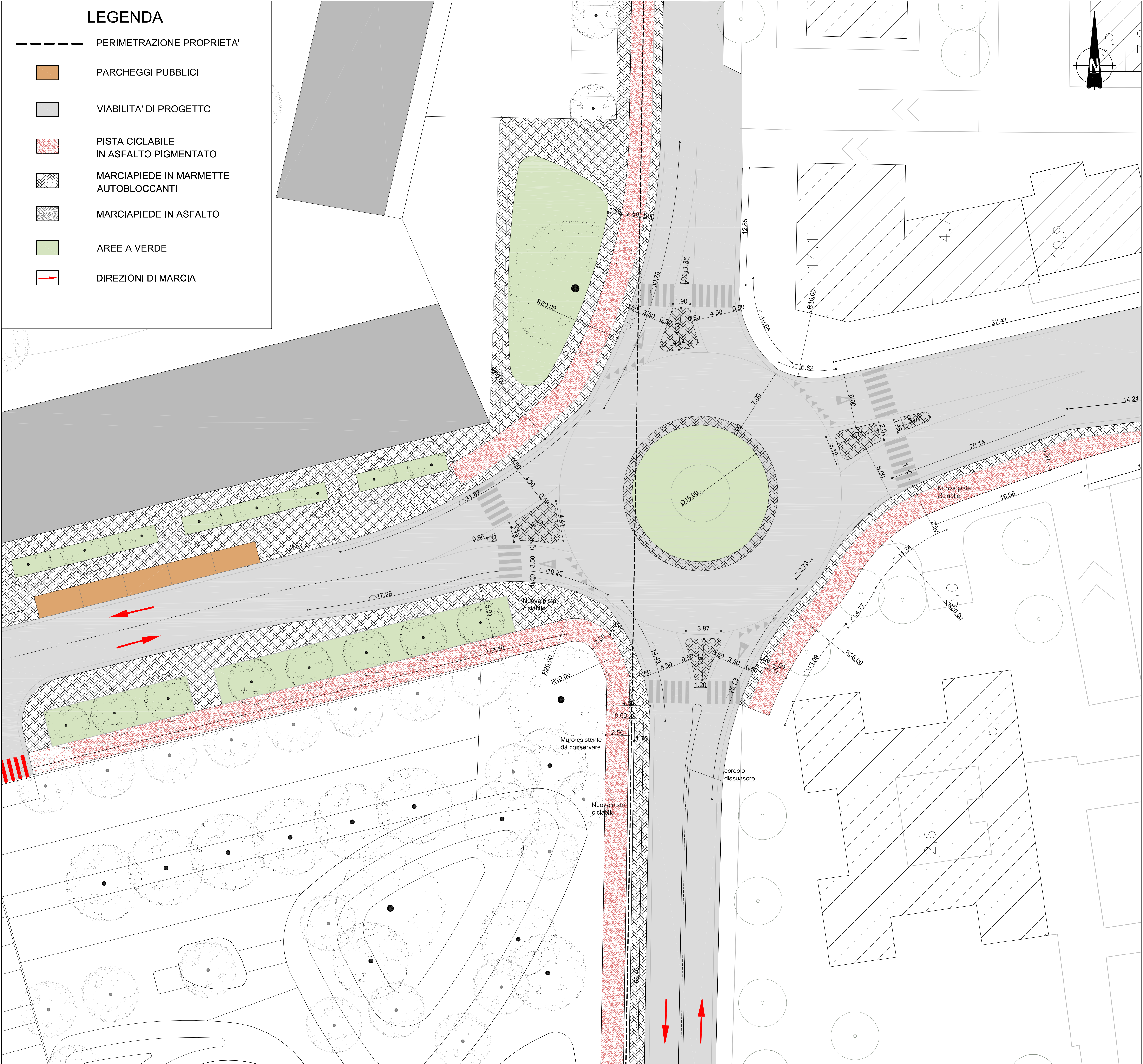
PIANTA ROTATORIA NORD scala 1:200
