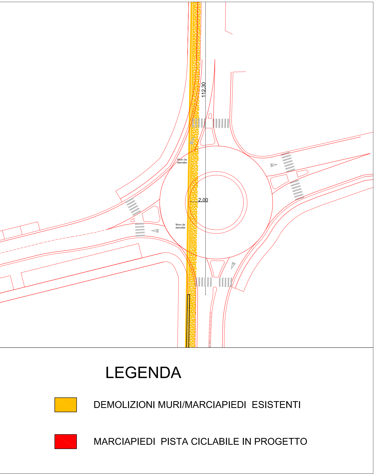
PIANTA ROTATORIA NORD scala 1:500 sovrapposizione nuovi interventi/demolizioni
