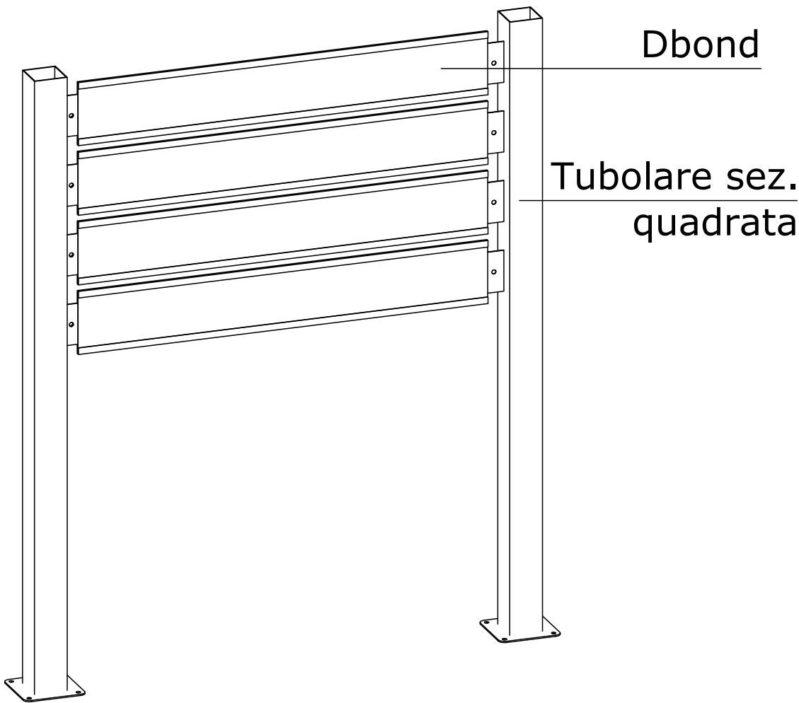
Assonometria
