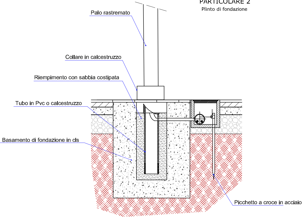
PARTICOLARE 2 Plinto di fondazione
