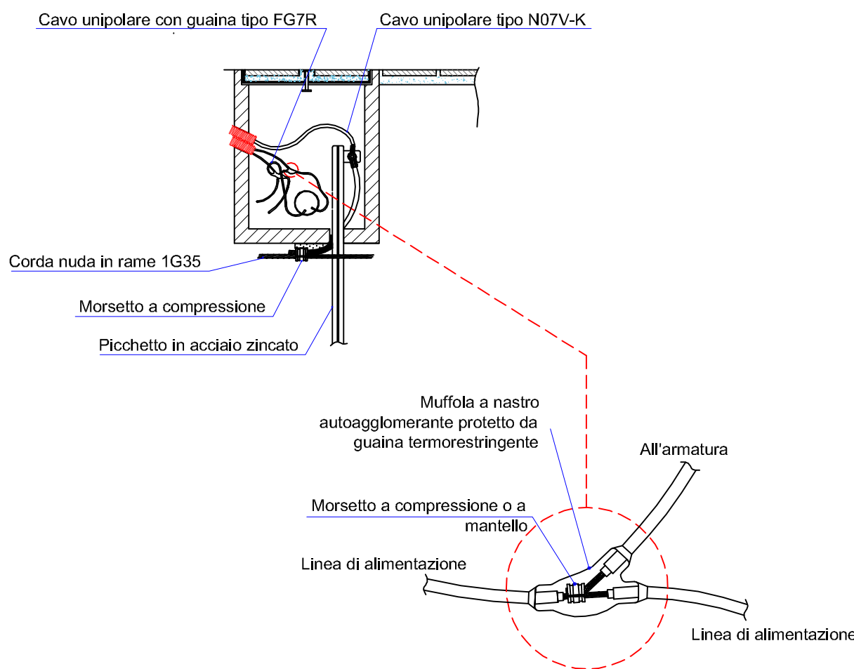
PARTICOLARE 3 Particolare di derivazione in pozzetto
