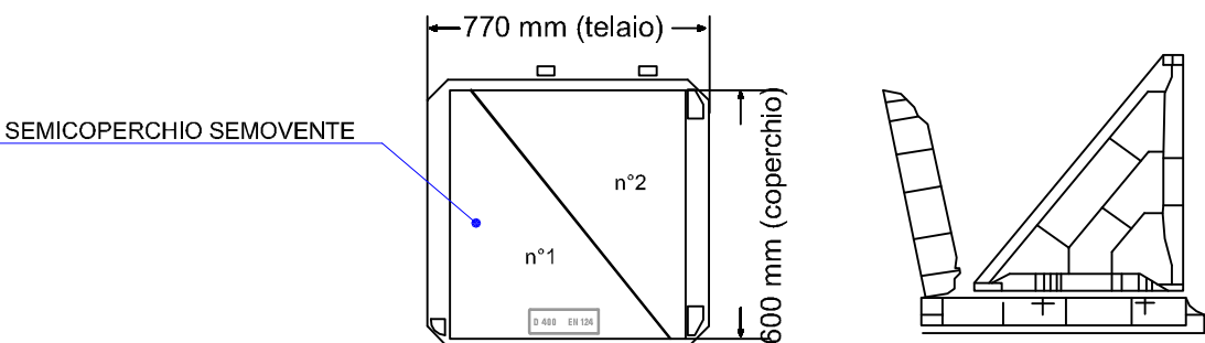
PARTICOLARE CHIUSINO IN GHISA Scala 1:40
