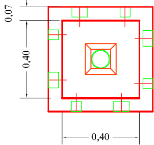
PARTICOLARE CHIUSINO IN GHISA Scala 1:40
