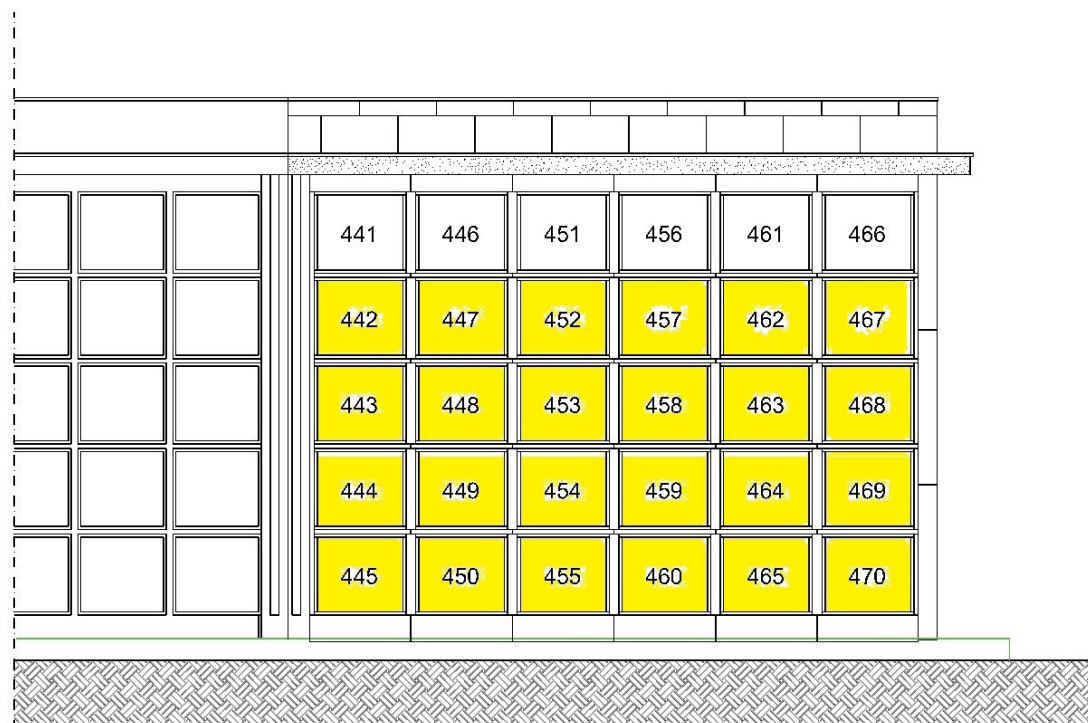
PROSPETTO FRONTALE
