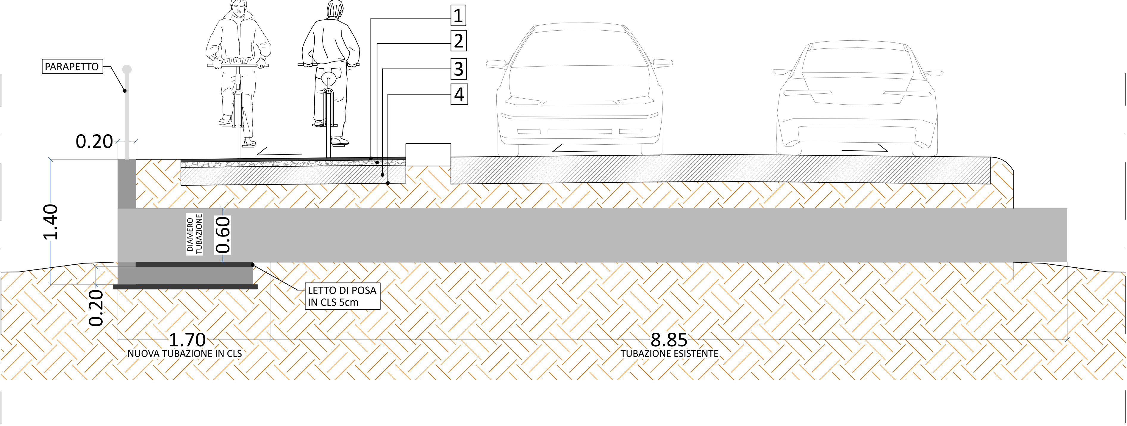
SEZIONE 3 PARTICOLARE COSTRUTTIVO scala 1:25
