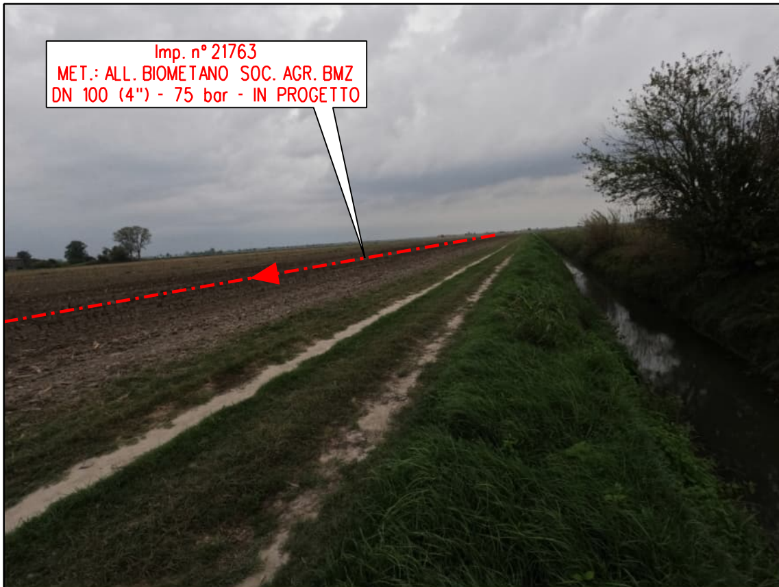
FOTO 3: VISTA PERCORRENZA CONDOTTA IN TERRENI AGRICOLI
