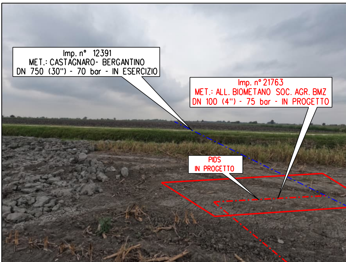
FOTO 4: VISTA AREA IMPIANTISTICA FINALE E MET. ESISTENTE
