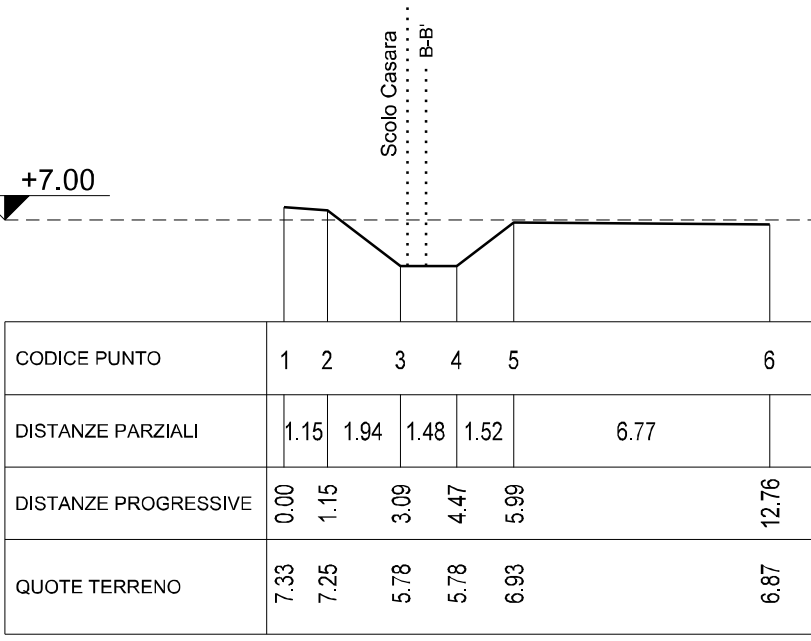
SEZIONE A-A' STATO DI FATTO scala 1:200
