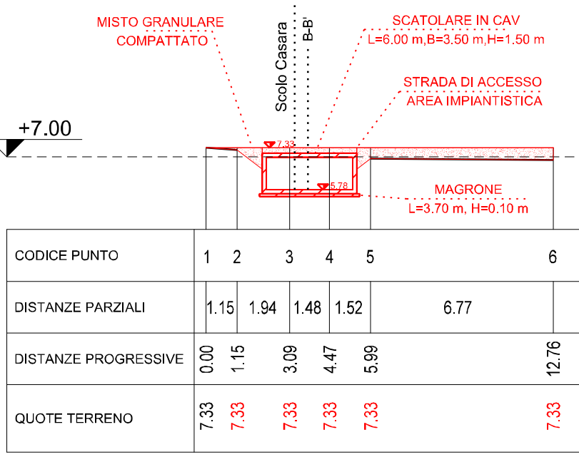
SEZIONE A-A' STATO DI PROGETTO scala 1:200
