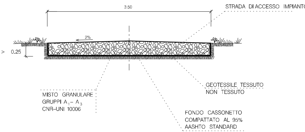
SEZIONE TIPO STRADA NON ASFALTATA scala 1:50
