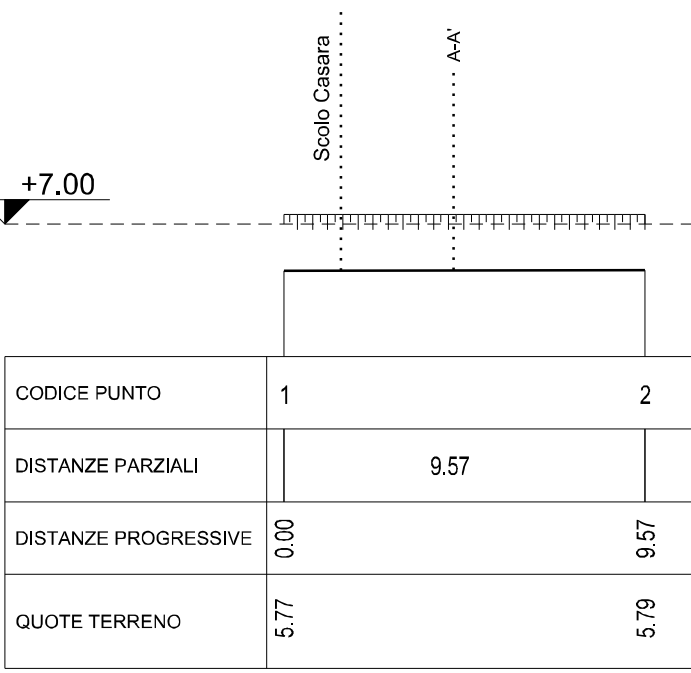
SEZIONE B-B' STATO DI FATTO scala 1:200
