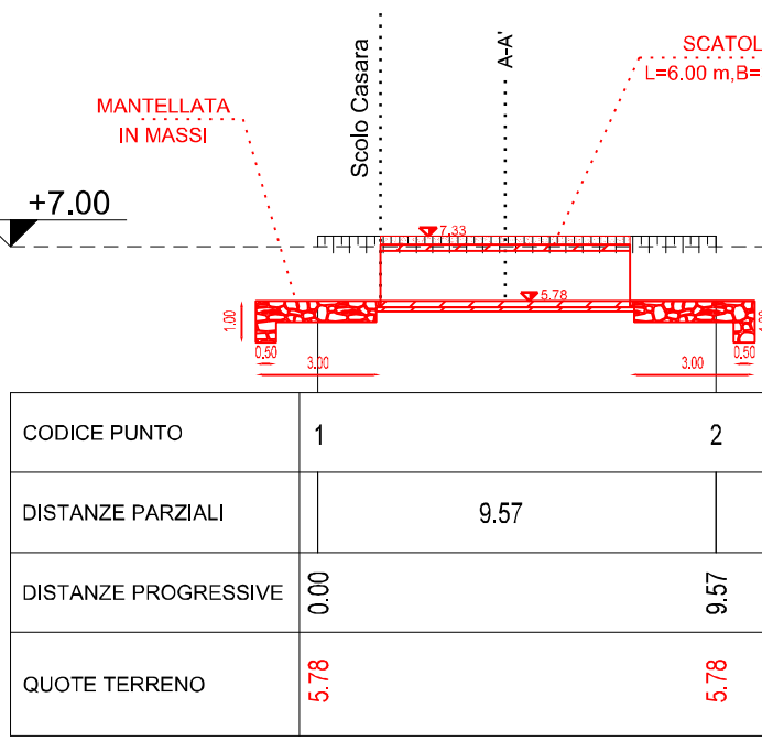
SEZIONE B-B' STATO DI PROGETTO scala 1:200
