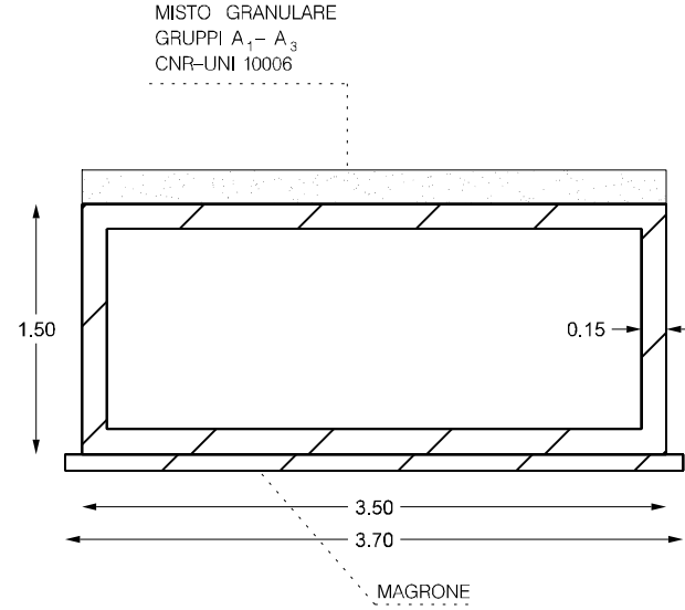
SEZIONE SCATOLARE scala 1:50
