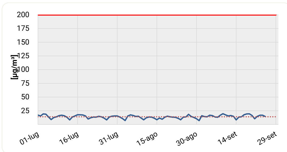
Figura 5: Concentrazioni medie giornaliere di NO 2 (Valore limite orario: 200 µg/m 3 ).
