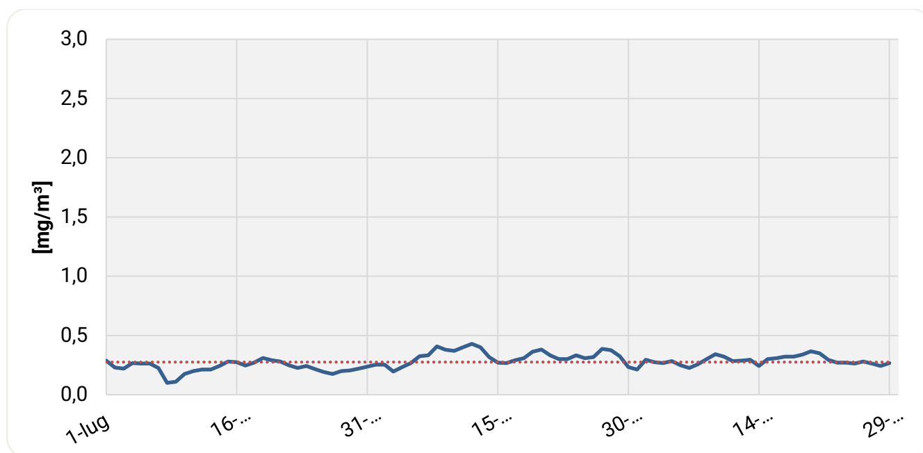
Figura 4: Concentrazioni medie giornaliere di CO (Valore limite 10 mg/m 3 ).
