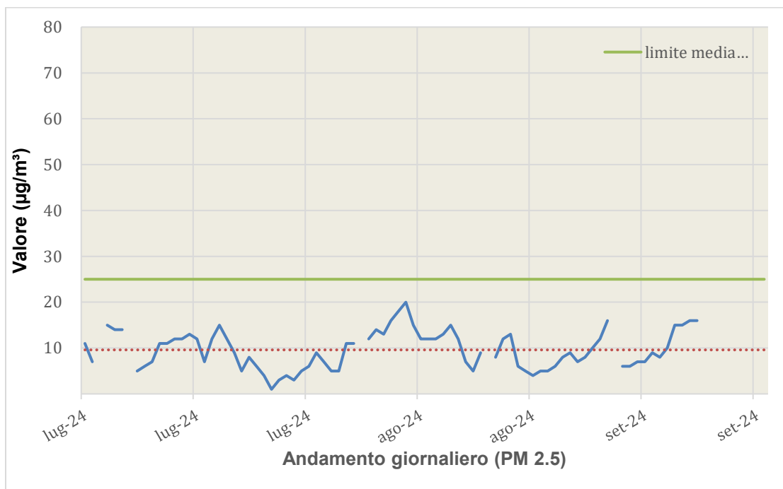
Figura 3: Concentrazioni giornaliere di PM2.5 (Valore limite 25 \mu\text{g}/\text{m}^3 su media annuale).
