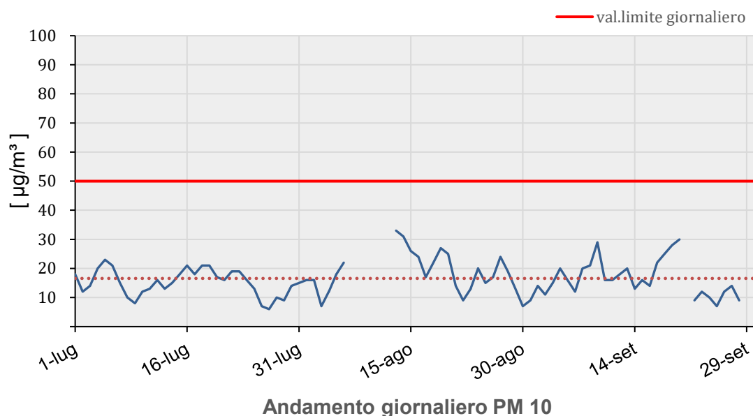
Figura 2: Concentrazioni giornaliere di PM10 (Valore soglia giornaliera: 50 \mu\text{g}/\text{m}^3 ).
