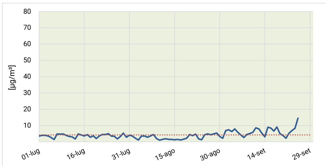
Figura 6: Concentrazioni medie giornaliere di NO
