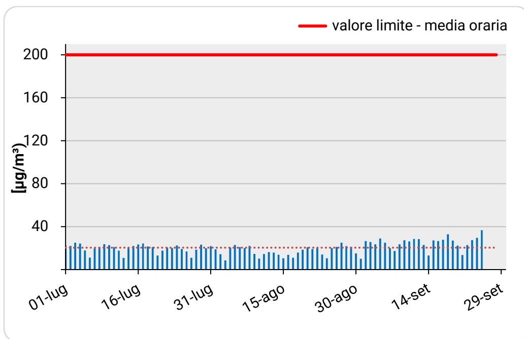
Figura 7: Concentrazioni medie giornaliere di NOx
