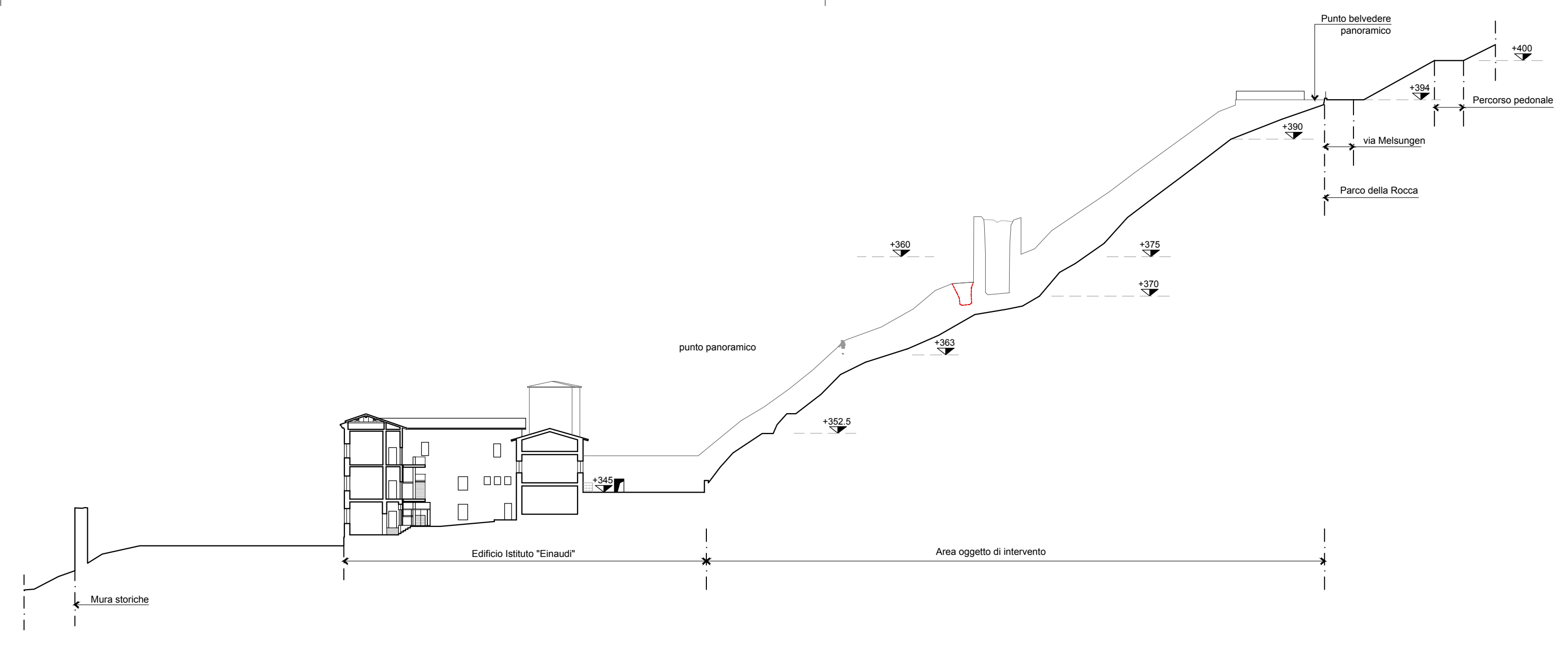
SEZIONE 1-1 SCALA 1:500
