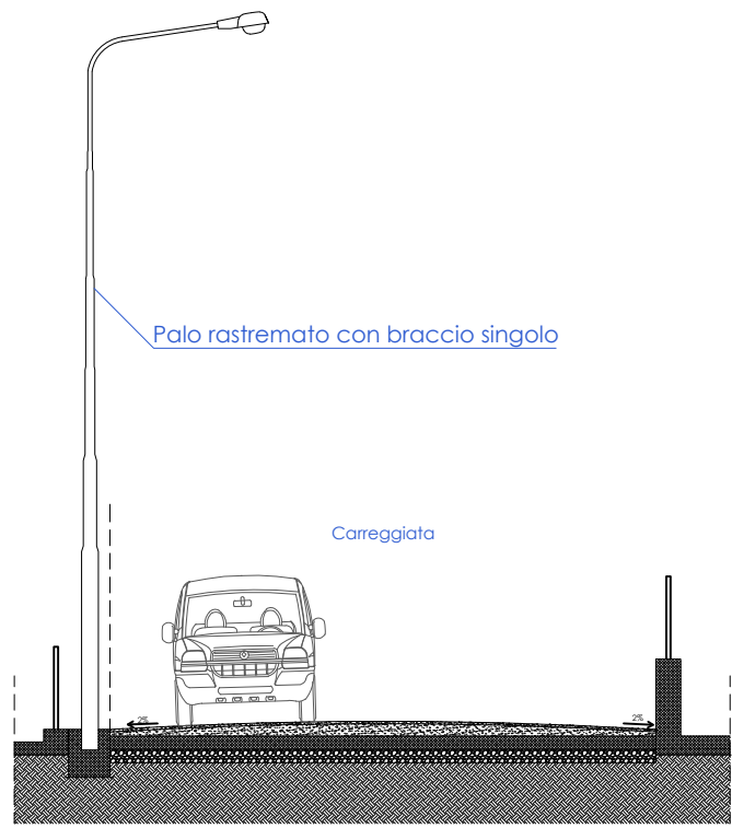
SEZIONE D
