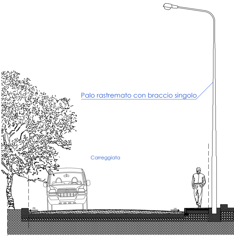
SEZIONE C
