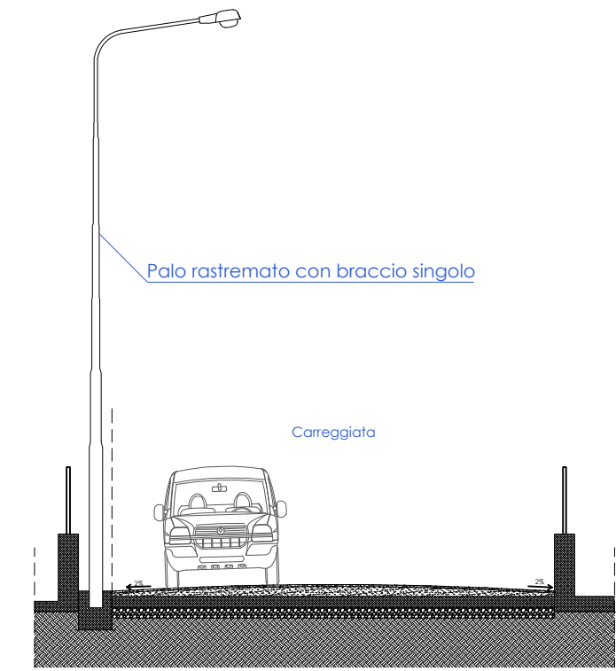
SEZIONE B
