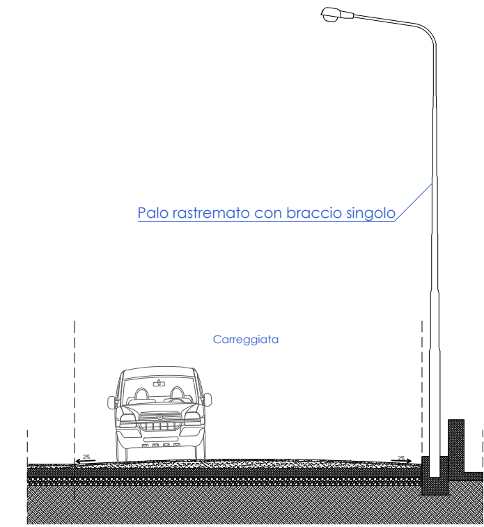
SEZIONE A
