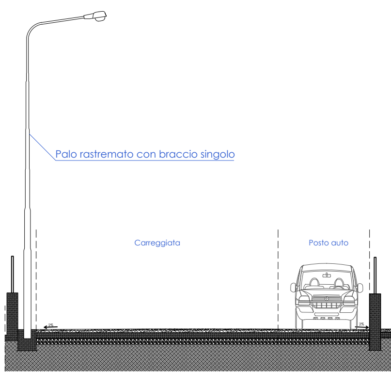
SEZIONE A
