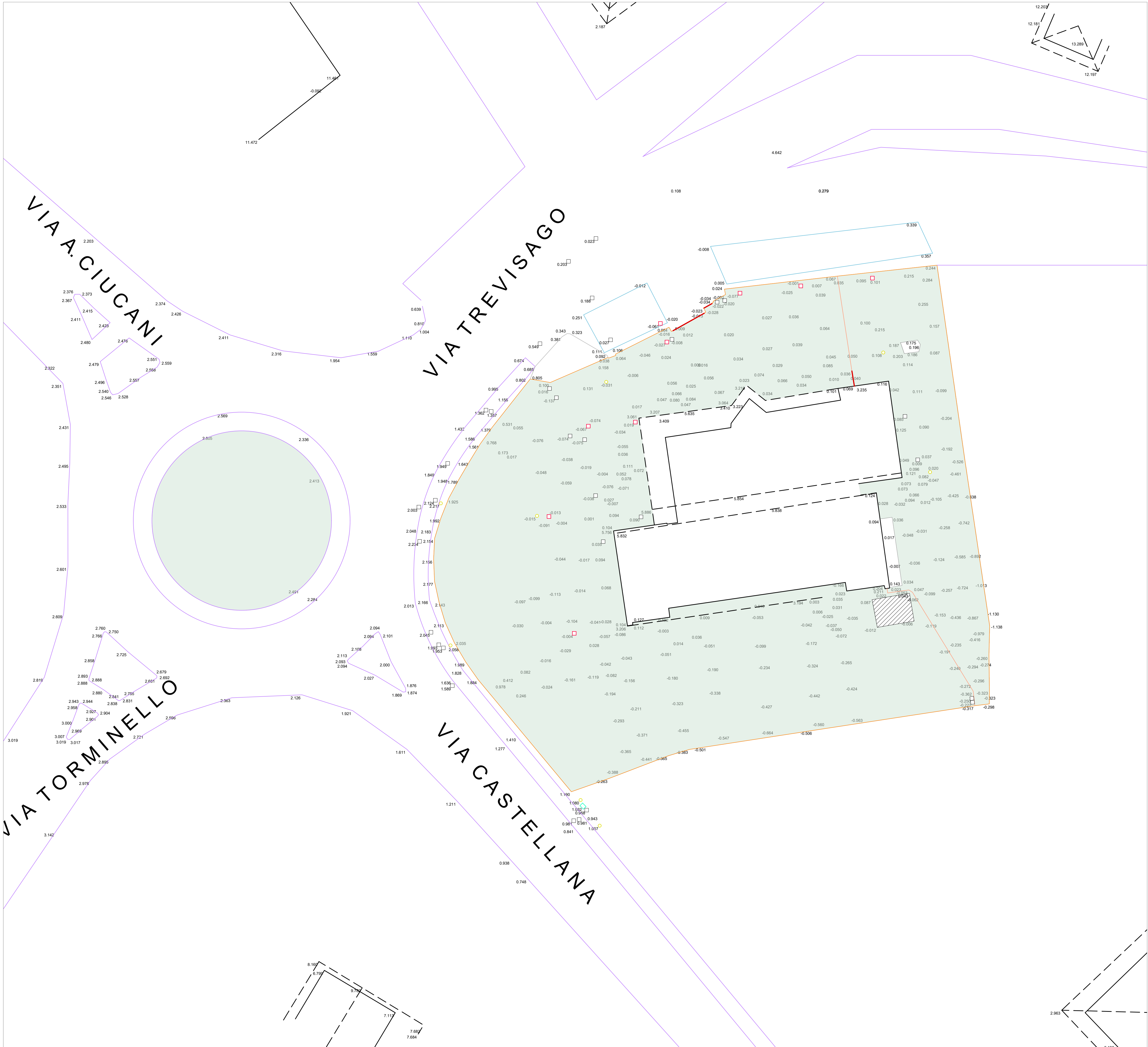
Rilievo topografico - 1:200
