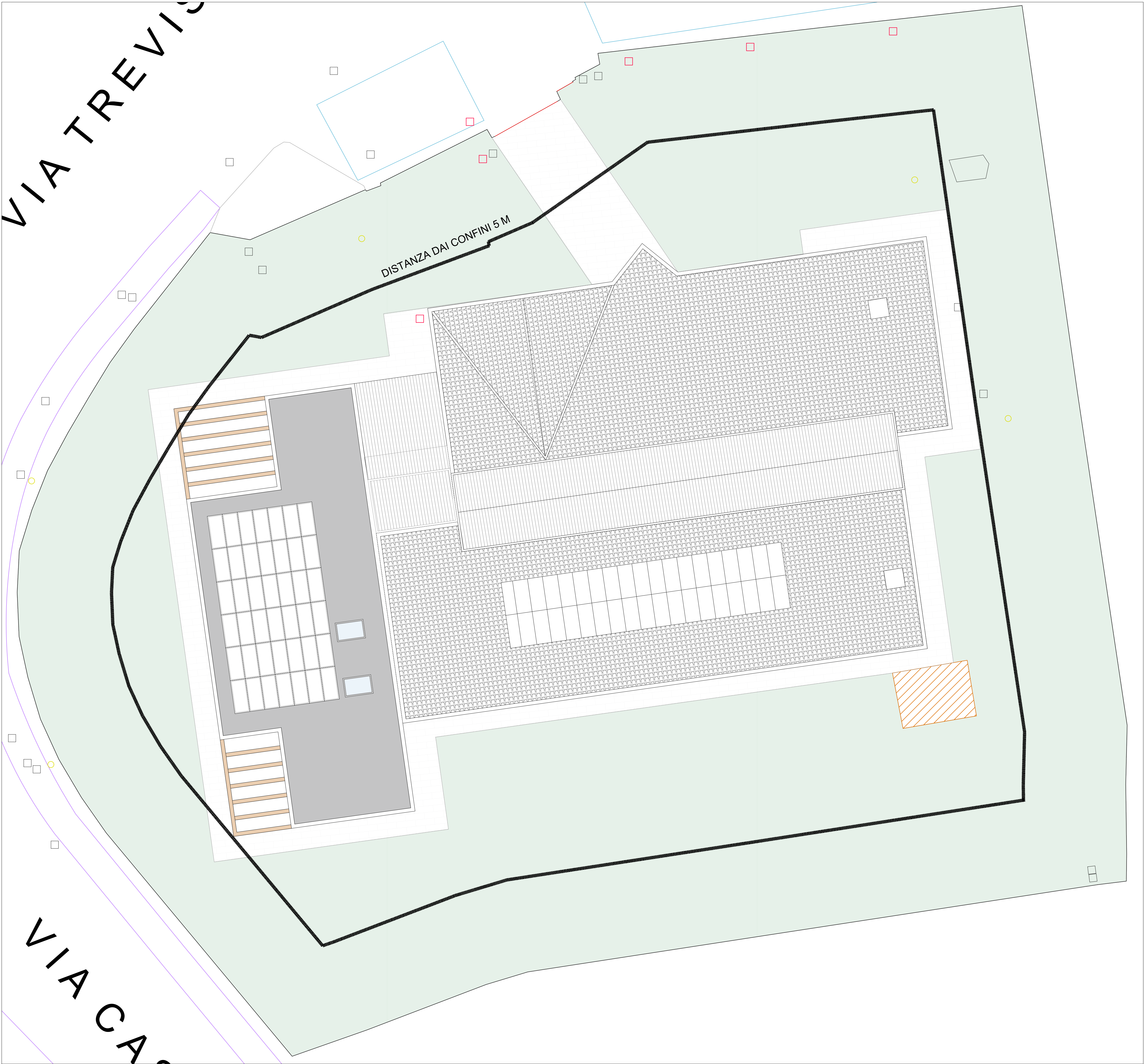
Pianta delle coperture_Stato di progetto - 1:100
