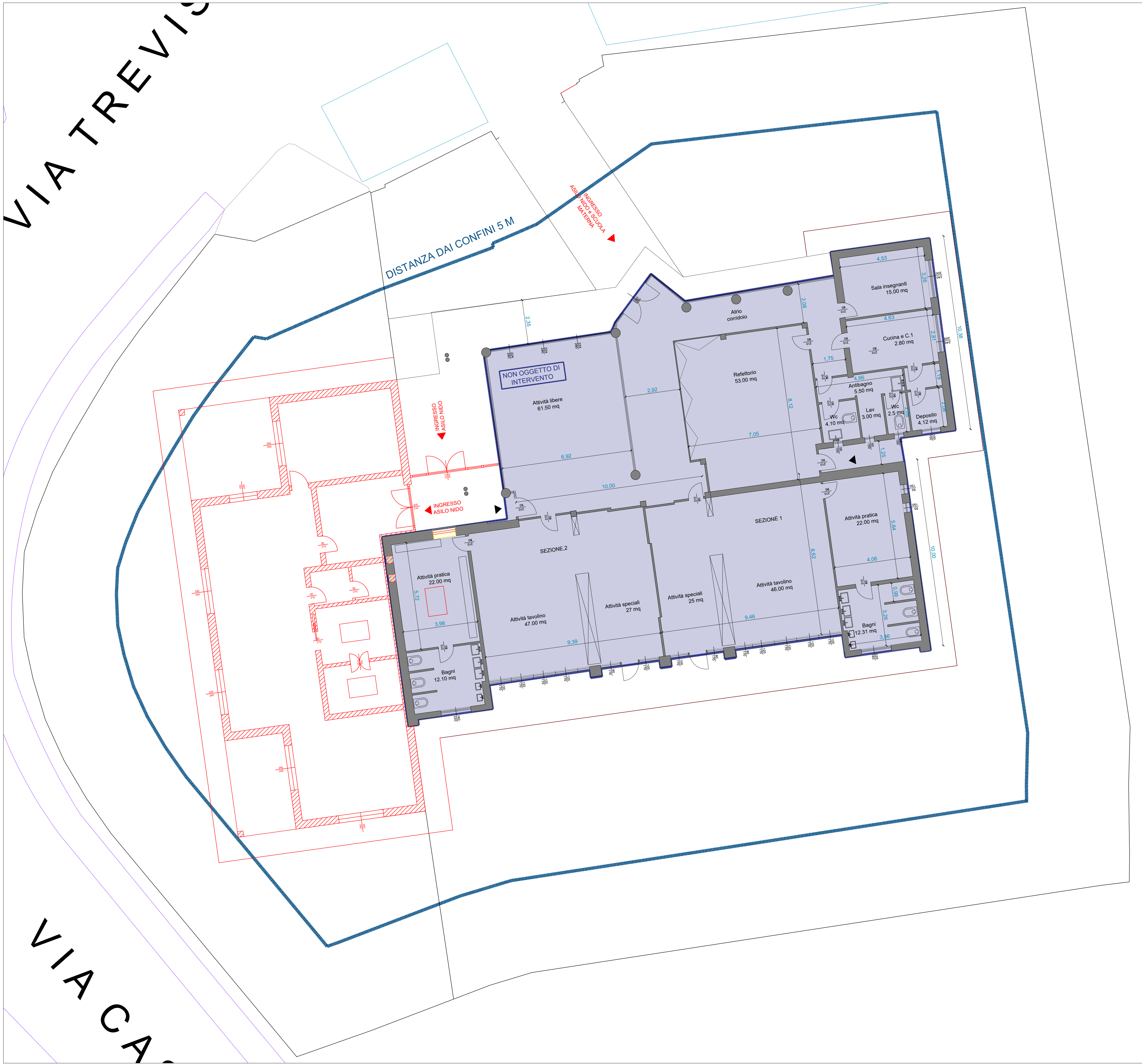
Attacco a terra_Stato di raffronto - 1:100
