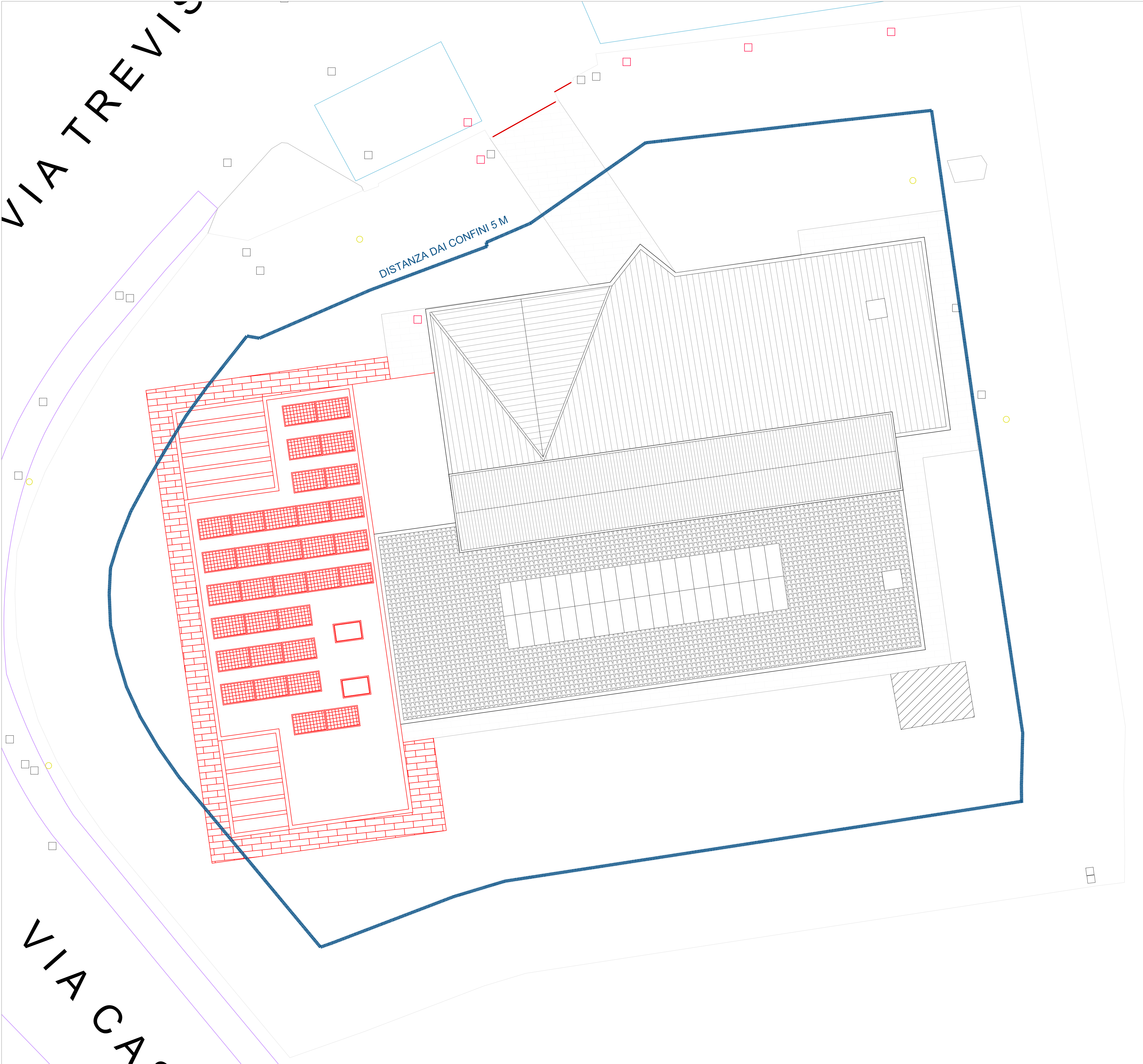
Pianta delle coperture_Stato di raffronto - 1:100
