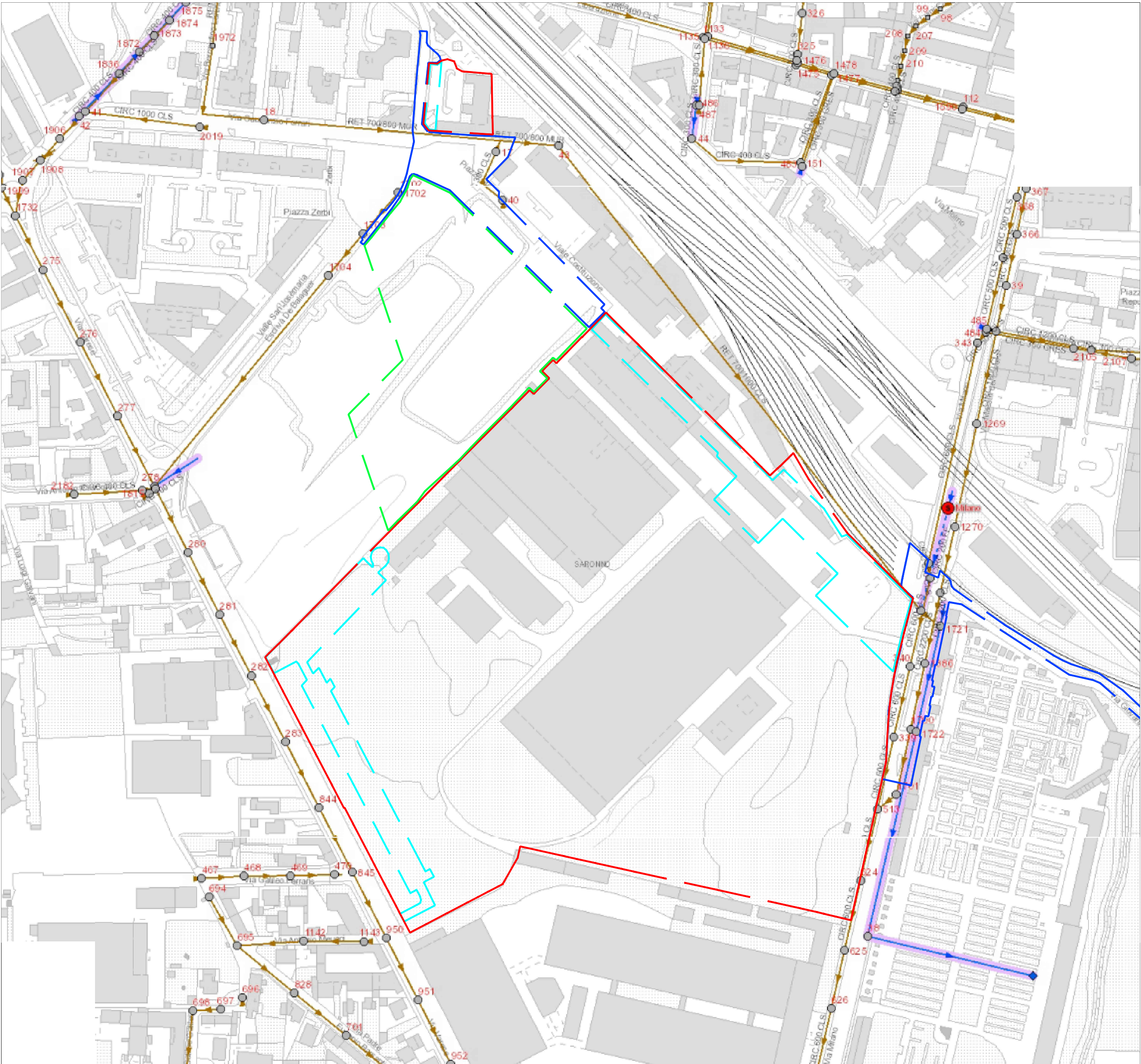
PLANIMETRIA STATO DI FATTO RETE FOGNARIA - ALFA- 05/04/2024
