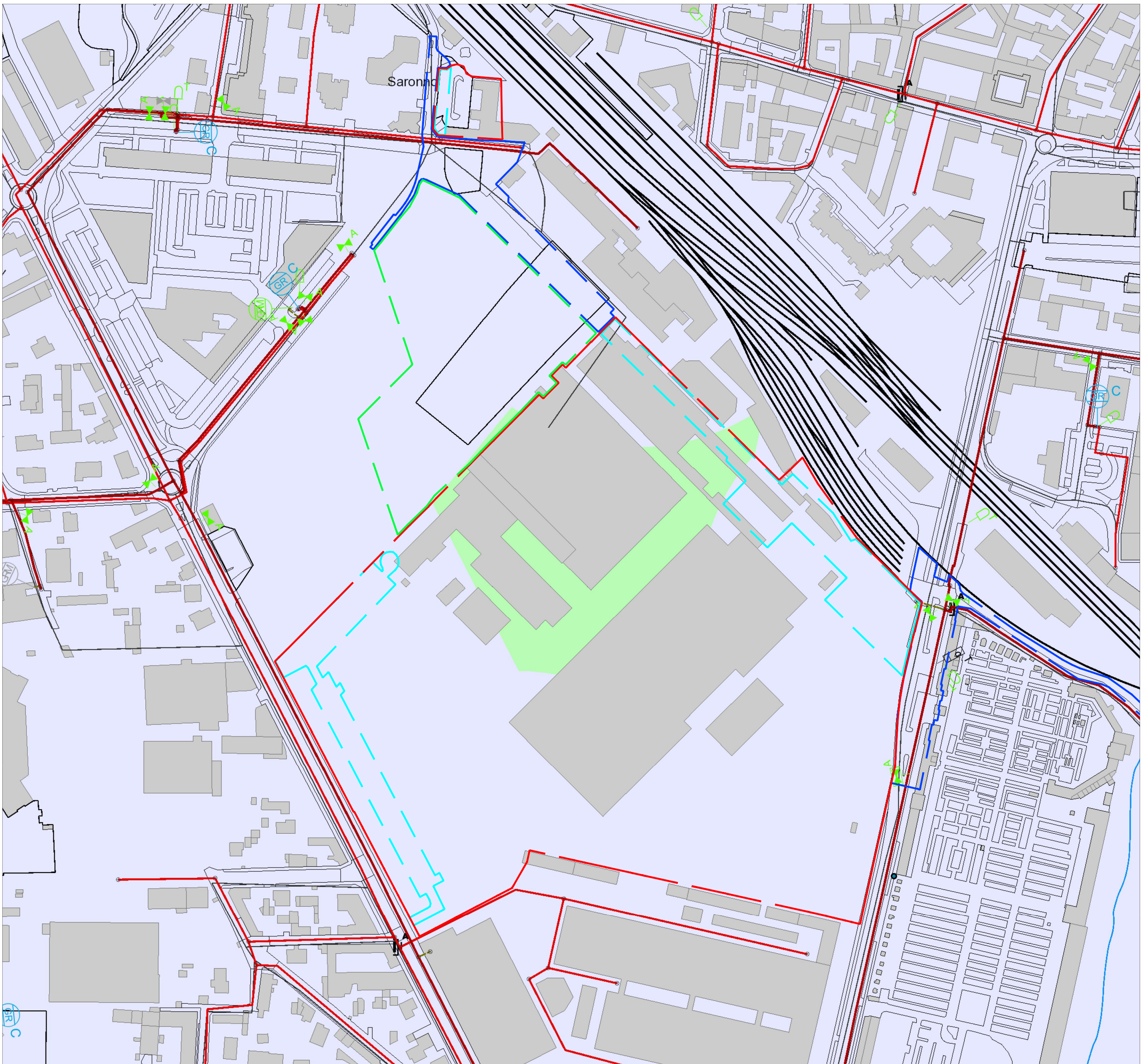
PLANIMETRIA STATO DI FATTO RETE GAS - 2i Rete Gas- 21/03/2024
