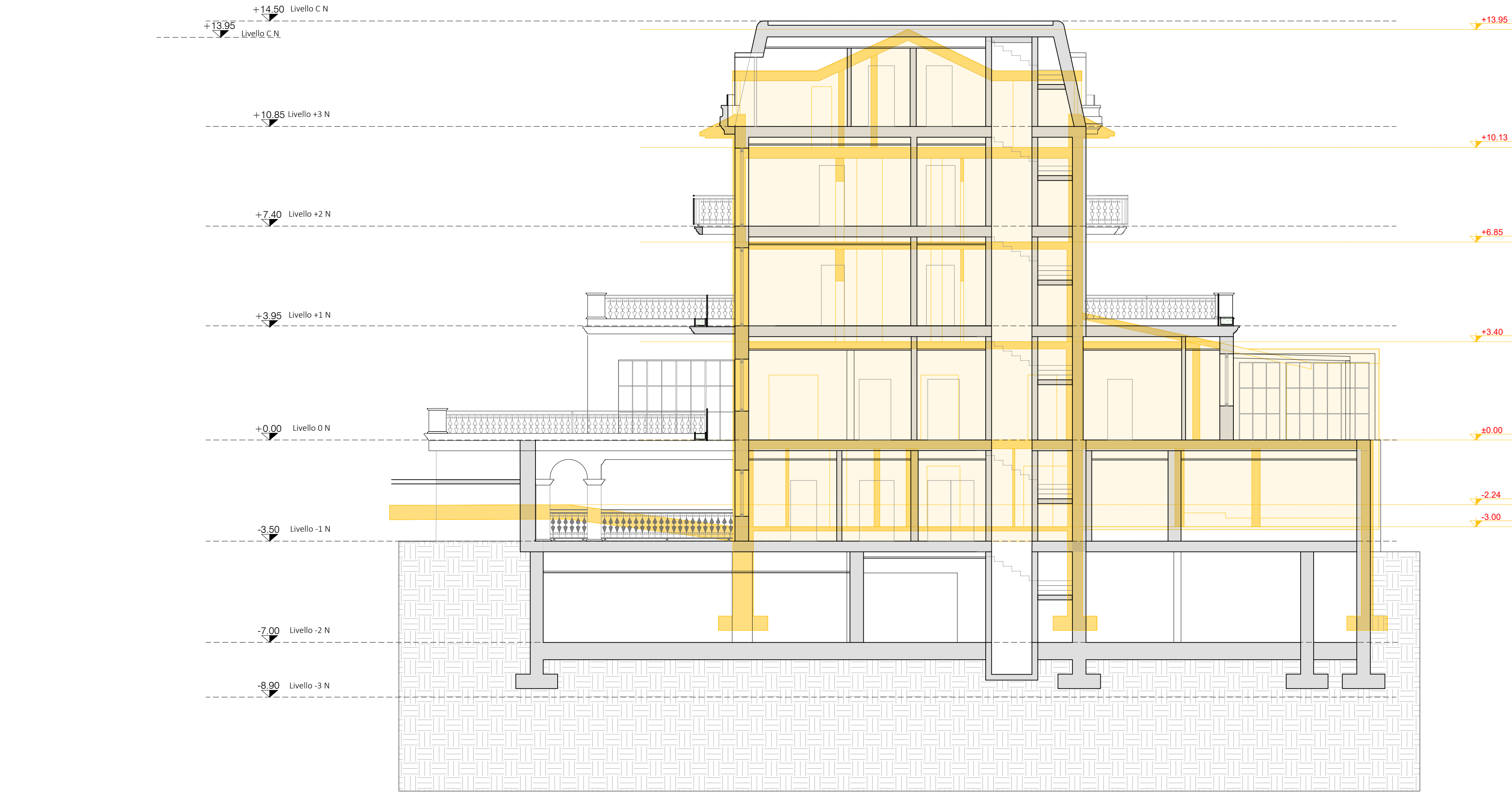
Prospetto est
