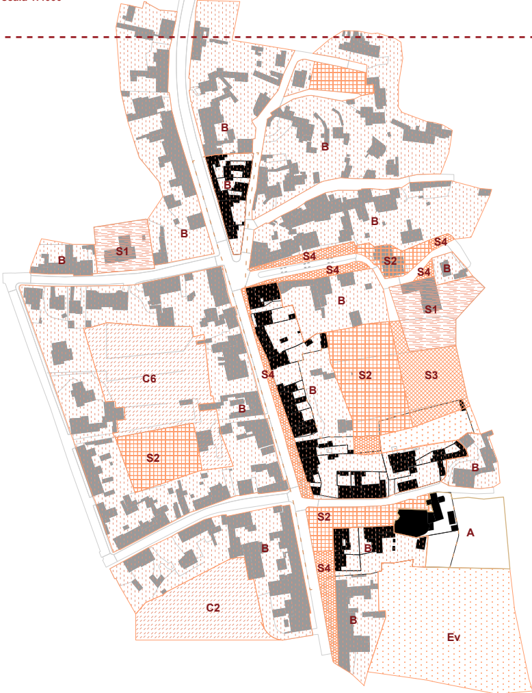
Areofotogrammetrico scala 1:4000
