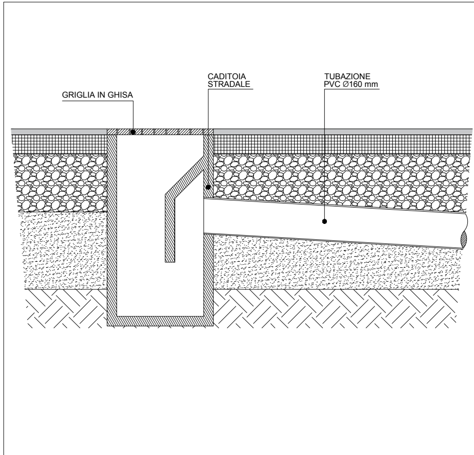
Caditoie stradale - Scala 1:20
