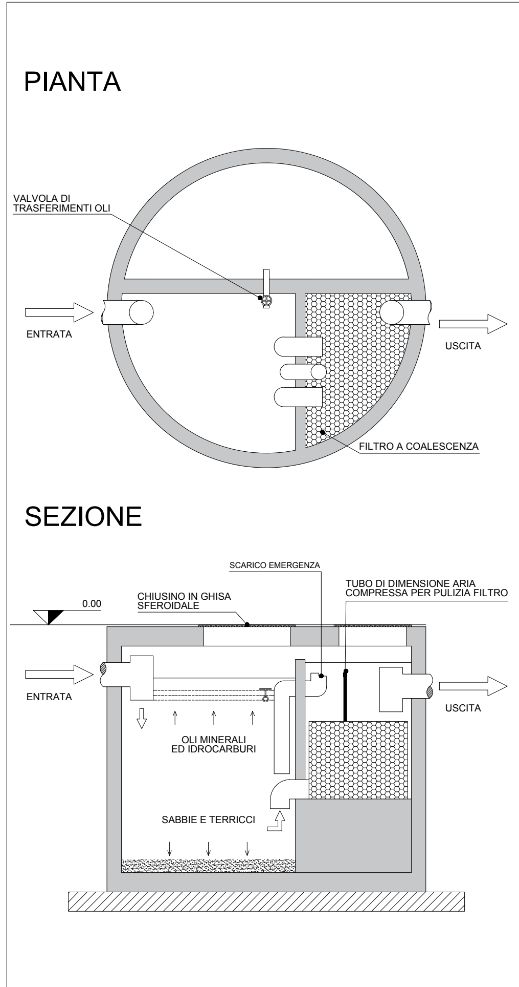
Disoleatore - Scala 1:20
