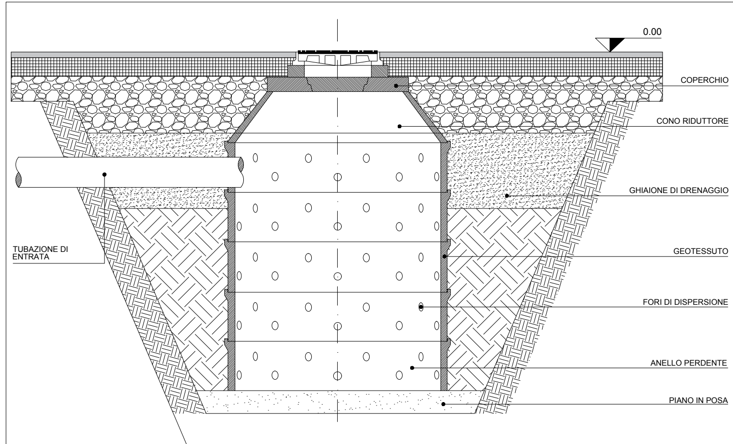
Pozzo perdenite - Scala 1:20
