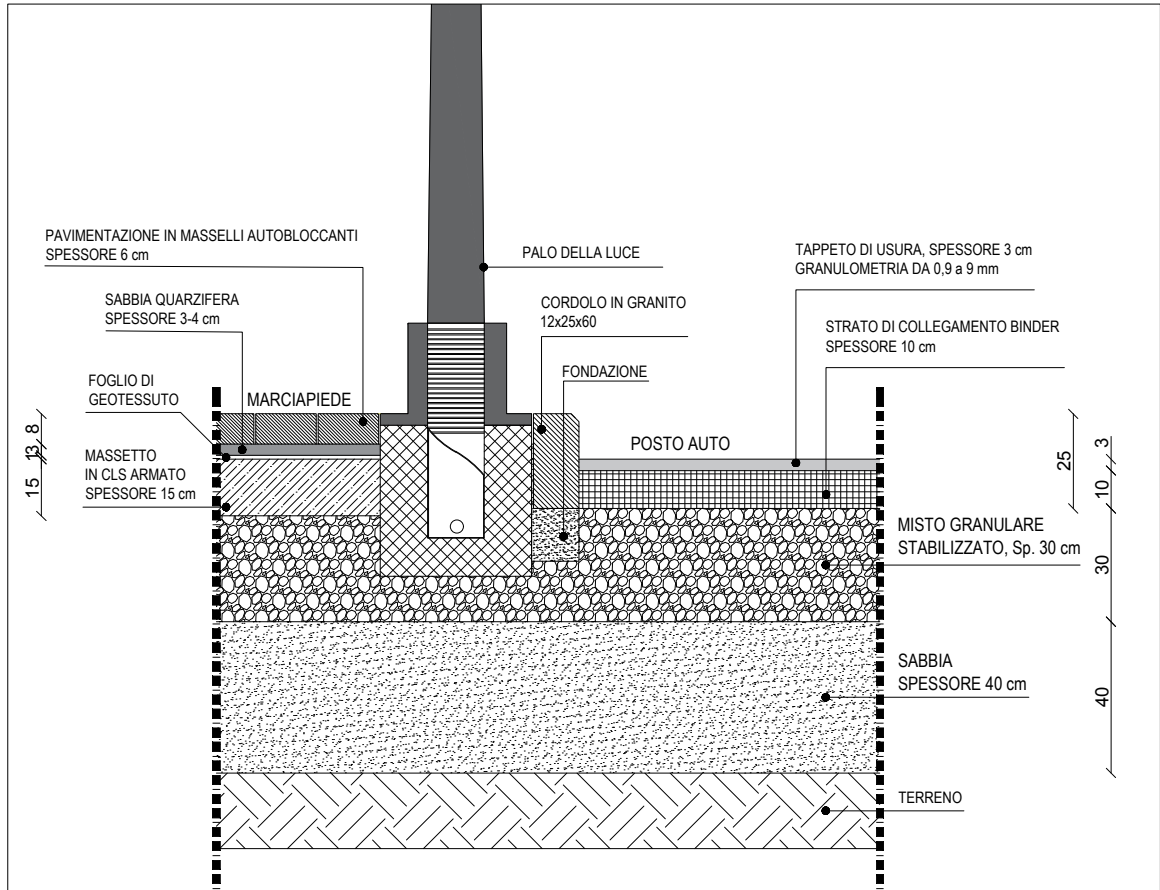
Delimitazione pedonale in corrispondenza dei posti auto - Scala 1:20
