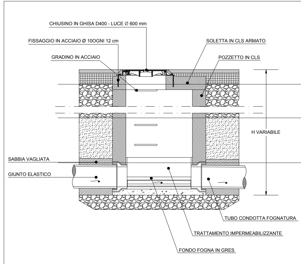
Pozzetto d'ispezione rete raccolta acque meteoriche - Scala 1:20
