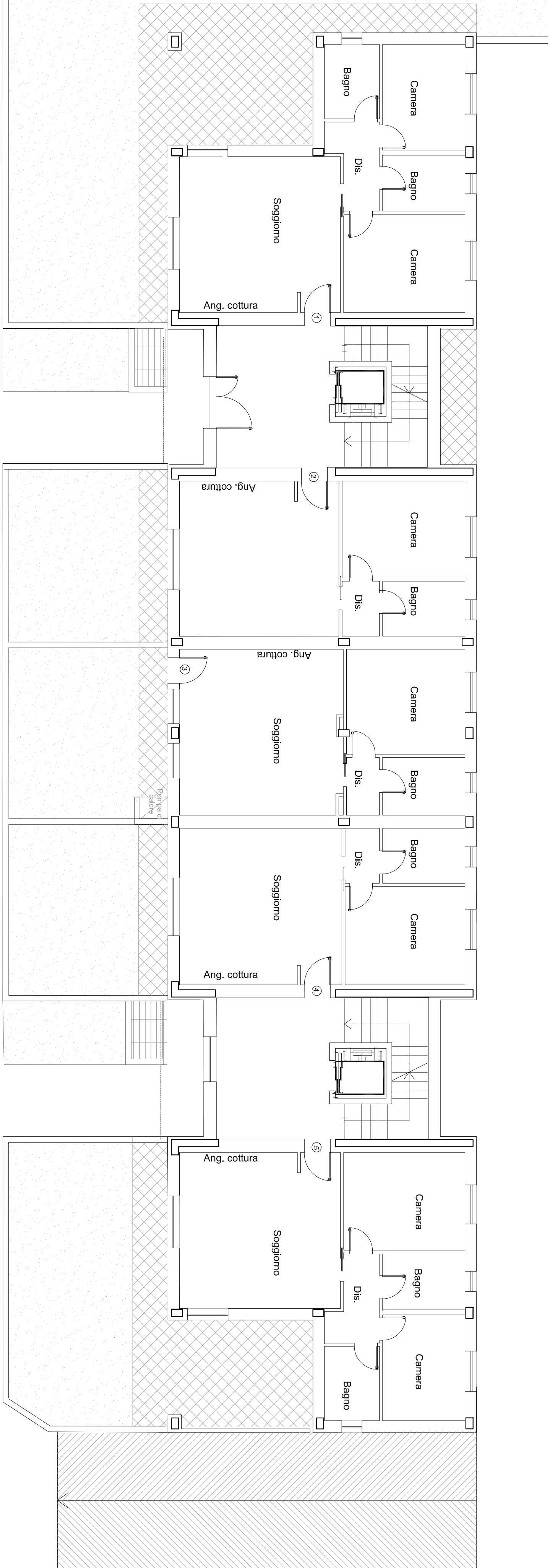
Pianta piano terra
