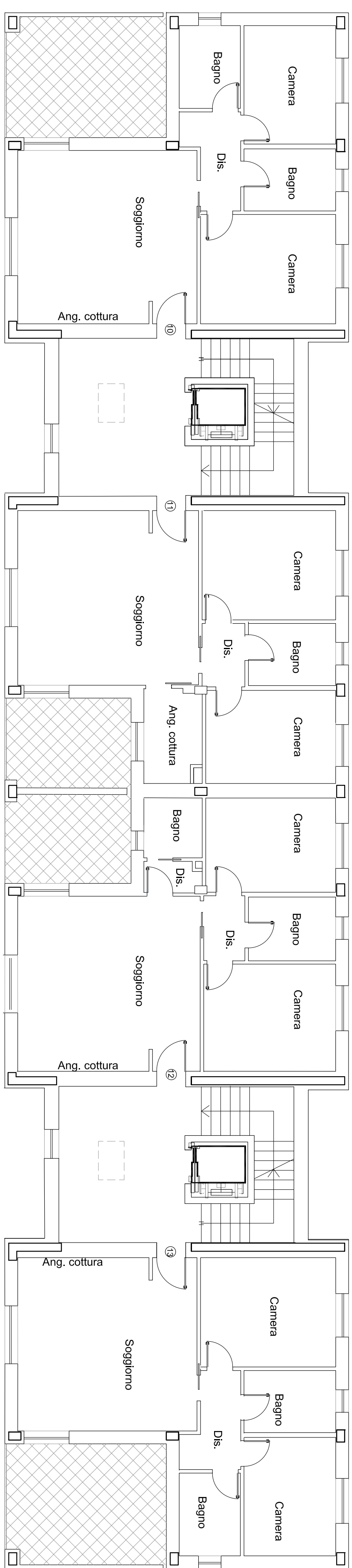
Pianta piano secondo
