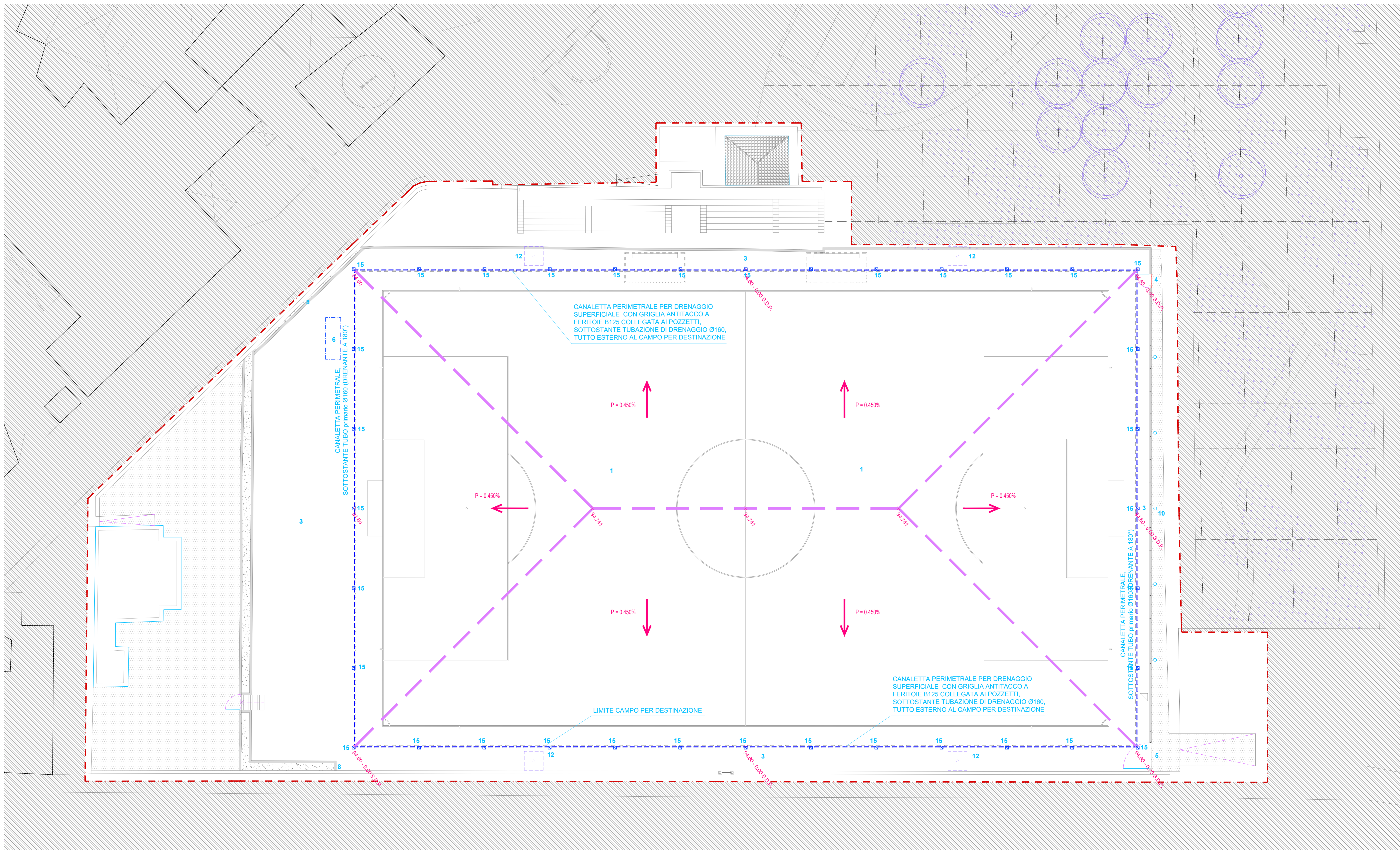
PLANIMETRIA GENERALE | INDICAZIONE DELLE PENDENZE DEL CAMPO PER DESTINAZIONE - SCALA 1:200
