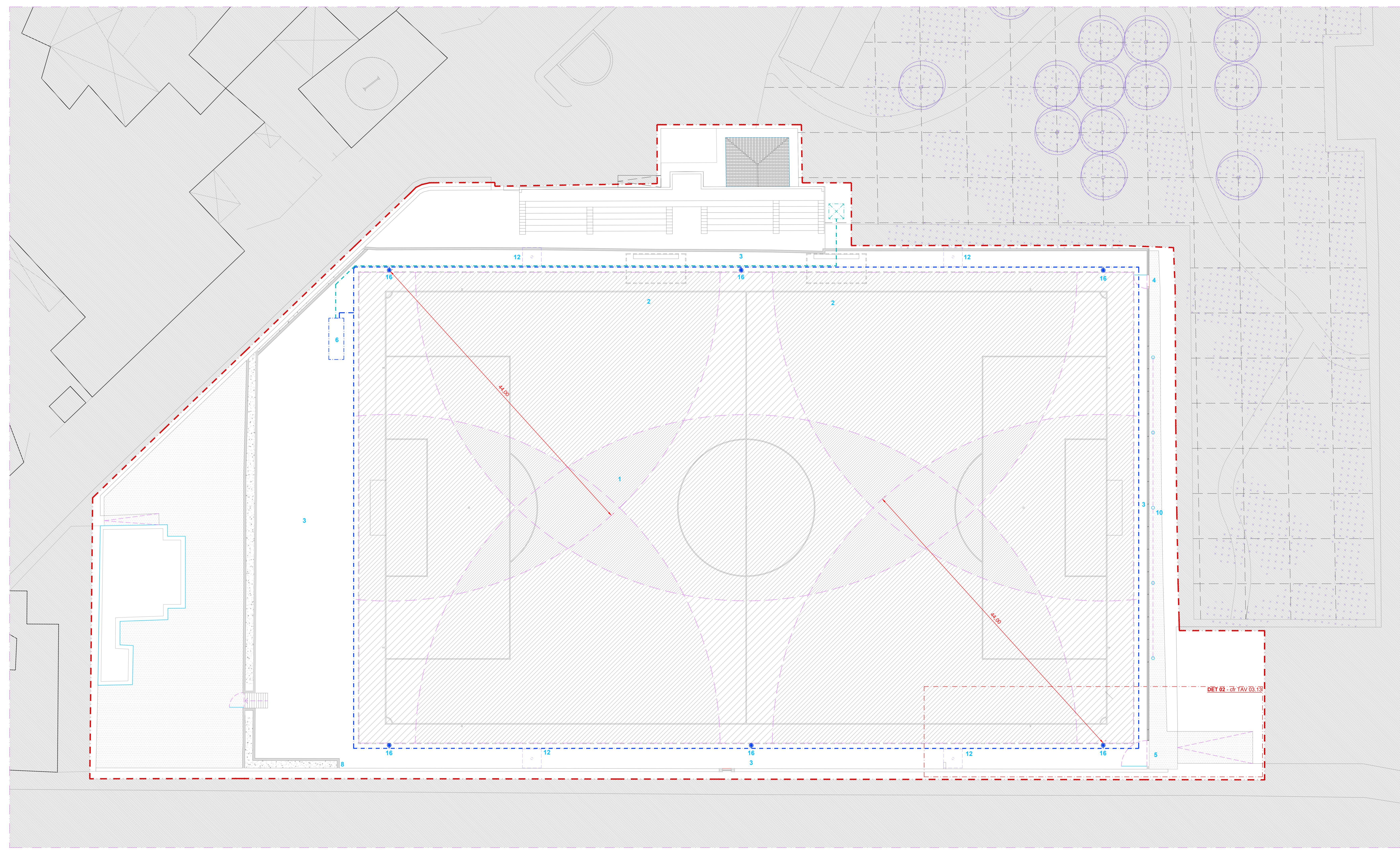
PLANIMETRIA GENERALE | SISTEMA DI IRRIGAZIONE CAMPO PER DESTINAZIONE - SCALA 1:200
