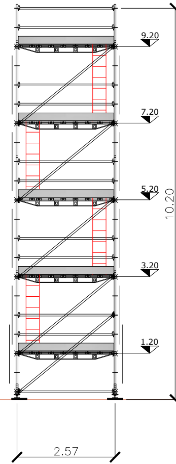
VISTA LATERALE
