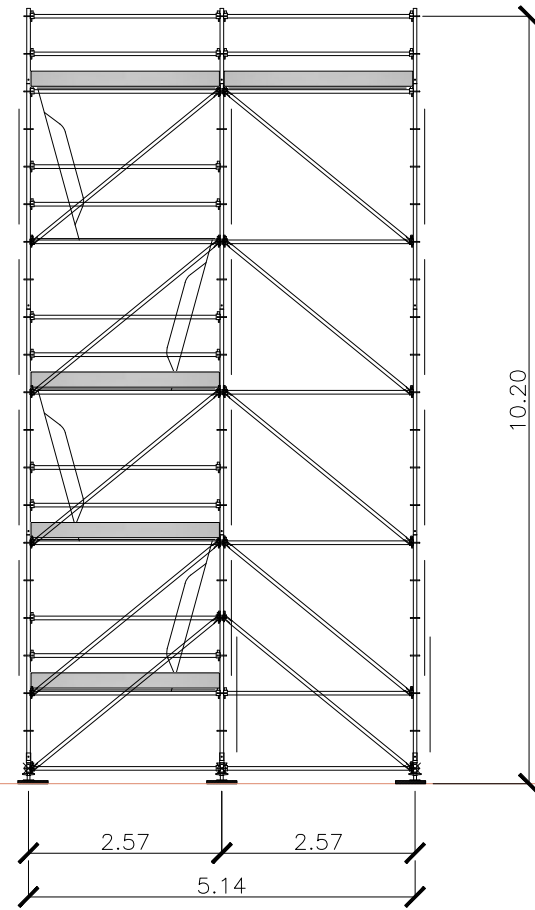
PROSPETTO FRONTALE
