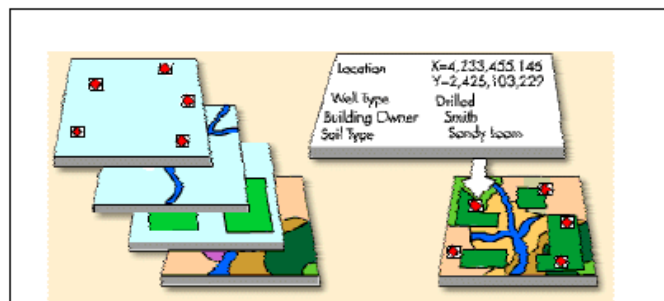
Immagine riguardante la tecnica di overlay in ambiente Geographical Information System, intesa come sovrapposizione di strati informativi al fine di costruire un unico strato informativo, definito "di sintesi".
