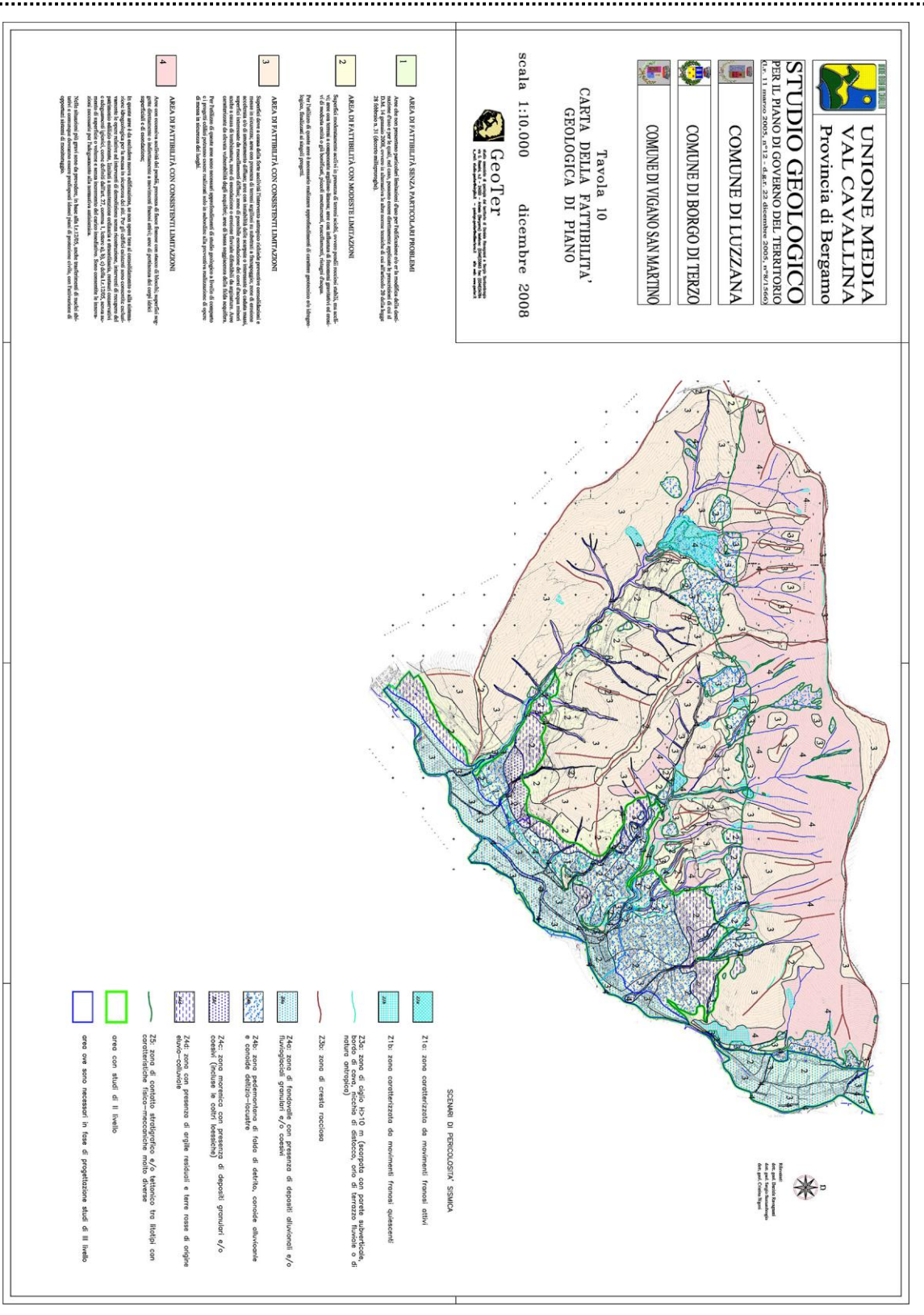
Figura 7. Componente geologica, idrogeologica e sismica: tavola 10 - Carta della fattibilità geologica
