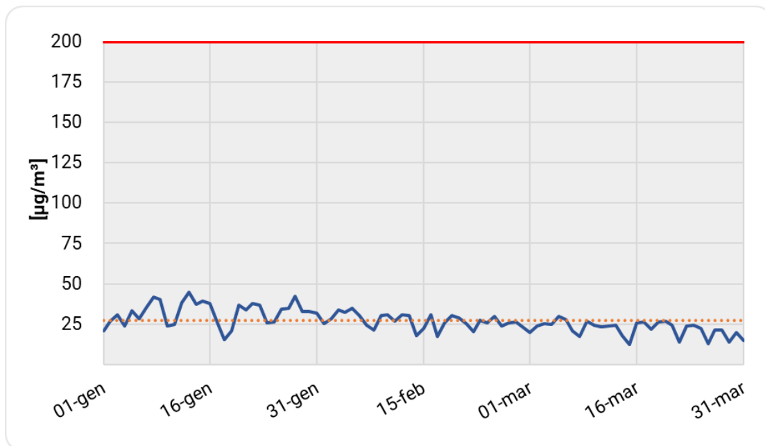
Figura 5: Concentrazioni medie giornaliere di NO 2 (Valore limite orario: 200 µg/m 3 ).
