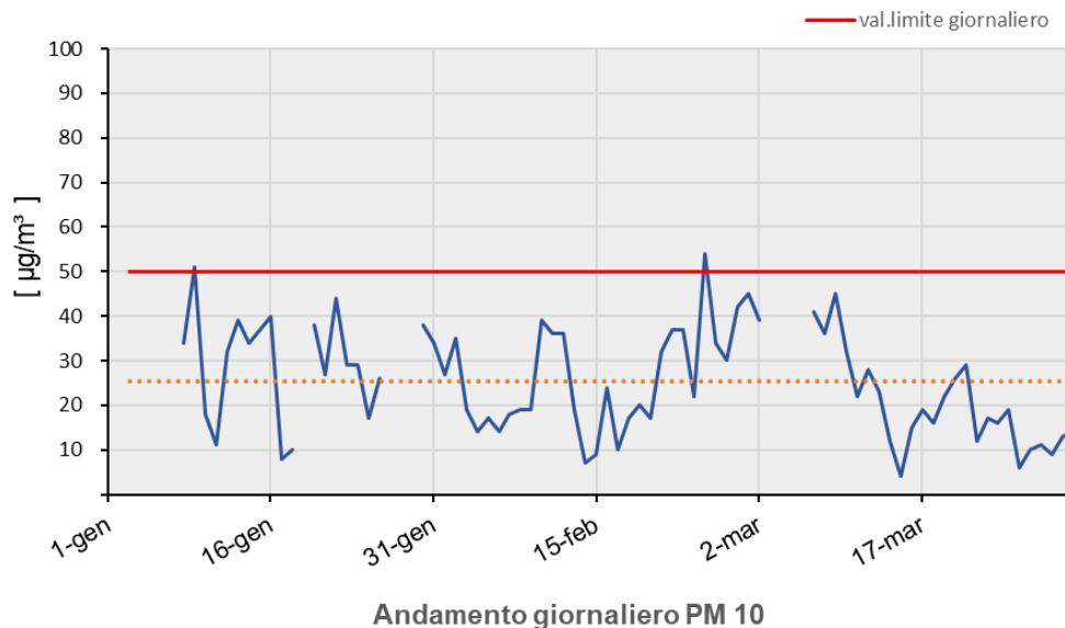
Figura 2: Concentrazioni giornaliere di PM10 (Valore soglia giornaliera: 50 µg/m³).
