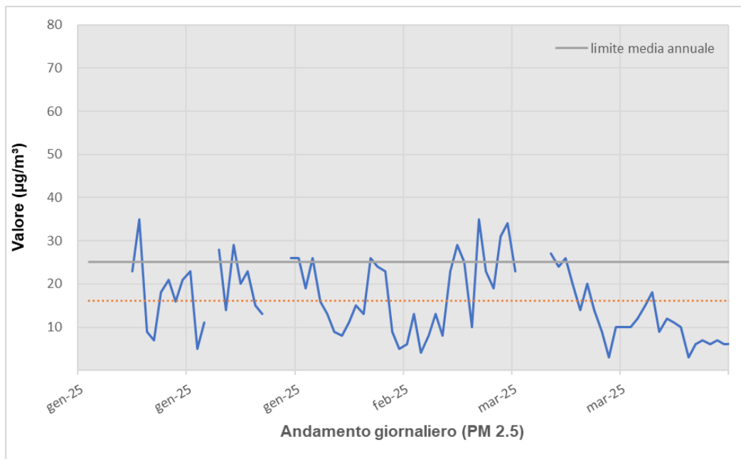
Figura 3: Concentrazioni giornaliere di PM2.5 (Valore limite 25 µg/m3 su media annuale).
