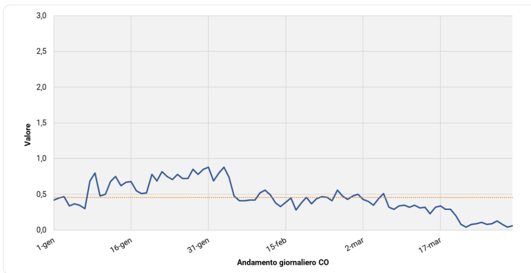
Figura 4: Concentrazioni medie giornaliere di CO (si noti che la line arancio ne tratteggiata rappresenta la media dei valori registrati)
