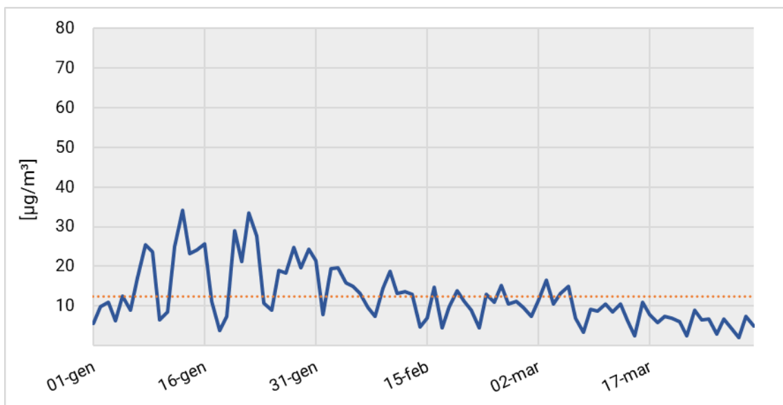
Figura 6: Concentrazioni medie giornaliere di NO
