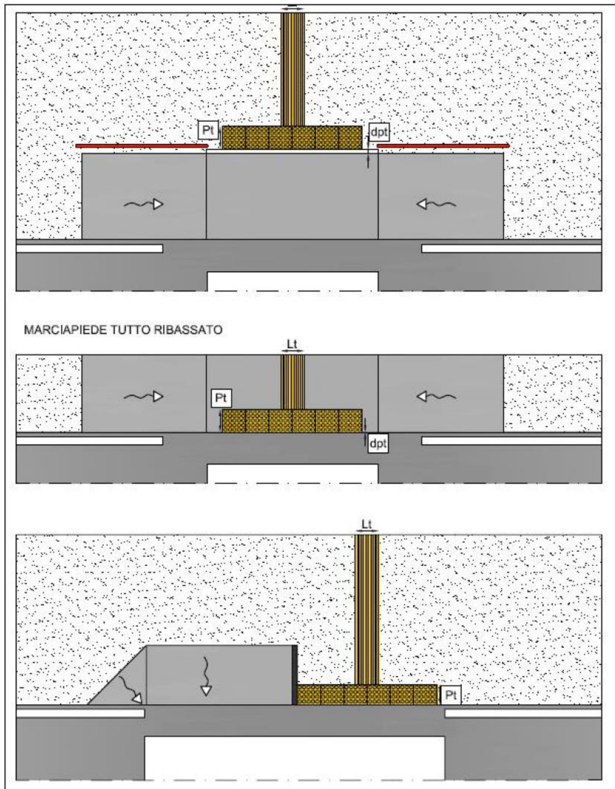
Figura 4-12 Pavimentazione tattile
