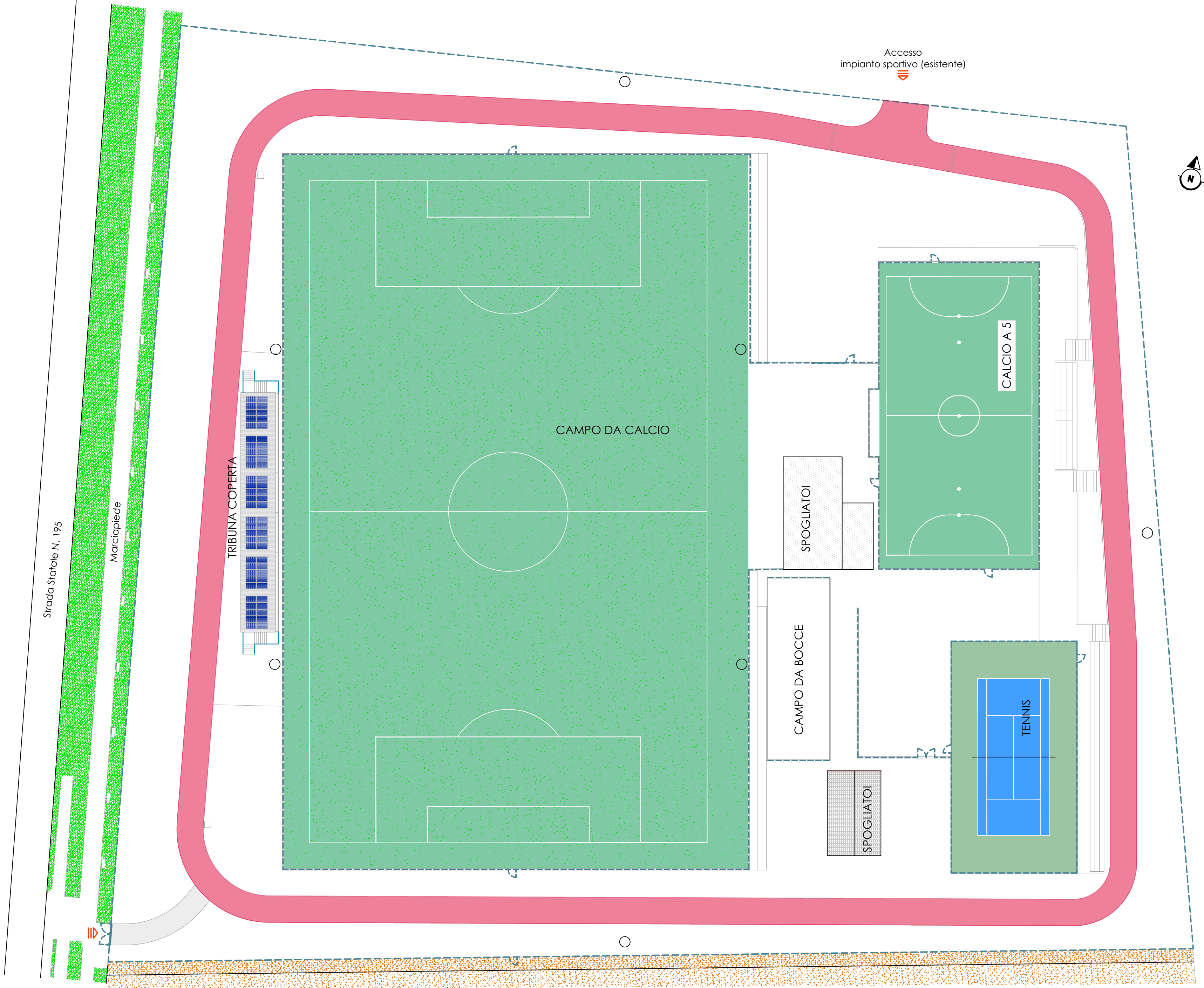
PLANIMETRIA GENERALE
