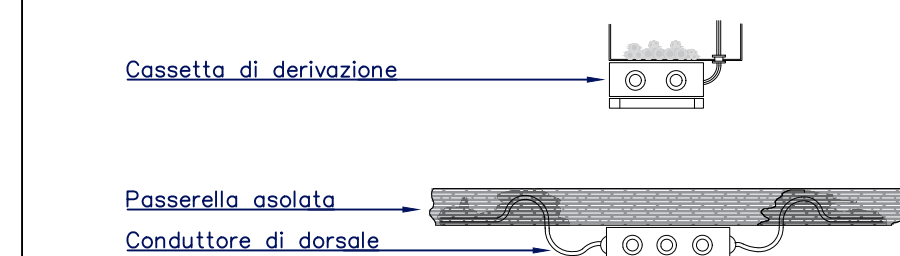
DETTAGLIO DERIVAZIONE IN CASSETTA DI DORSALE SU PASSERELLA DI DISTRIBUZIONE NEL CONTROSOFFIT STAFFATA A PARETE
