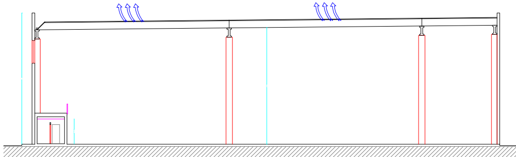
SEZIONE A-A' DI PROGETTO SCALA 1:200
