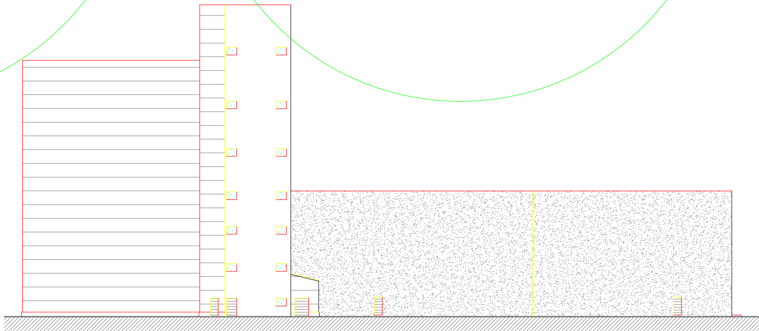
PROSPETTO EST DI PROGETTO SCALA 1:200
