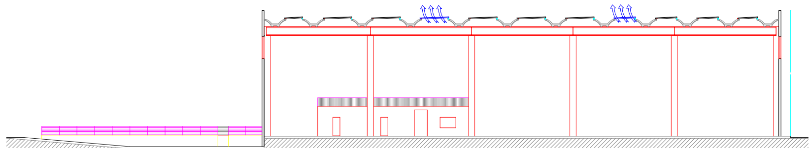
SEZIONE B-B' DI PROGETTO SCALA 1:200
