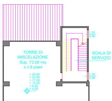
PIANTA PIANI INTEREDI DI PROGETTO SCALA 1:100
