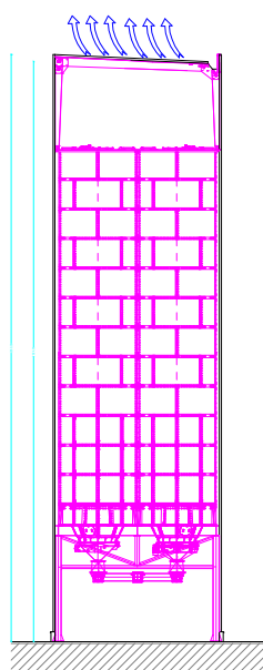
SEZIONE C-C' DI PROGETTO SCALA 1:200
