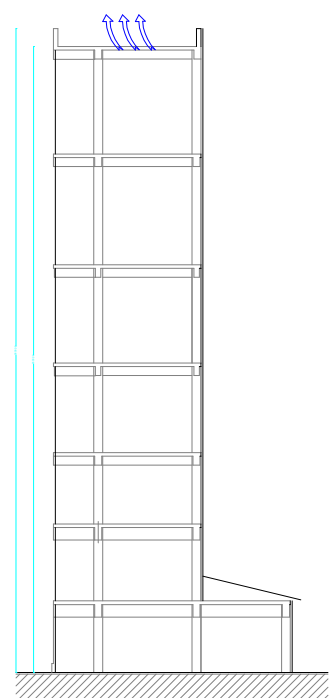
SEZIONE D-D' DI PROGETTO SCALA 1:200
