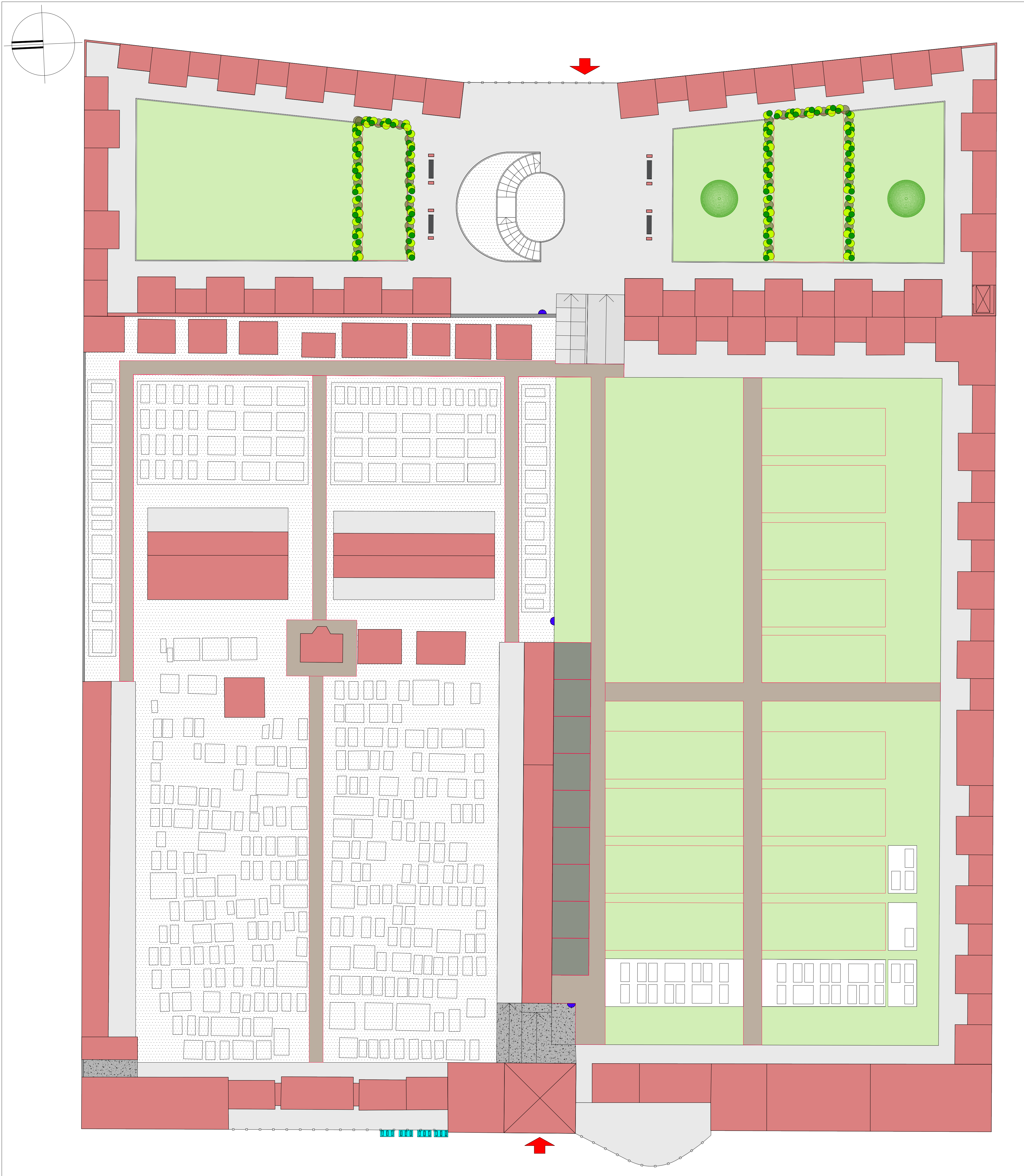
planimetria generale piano terra - scala 1:200
