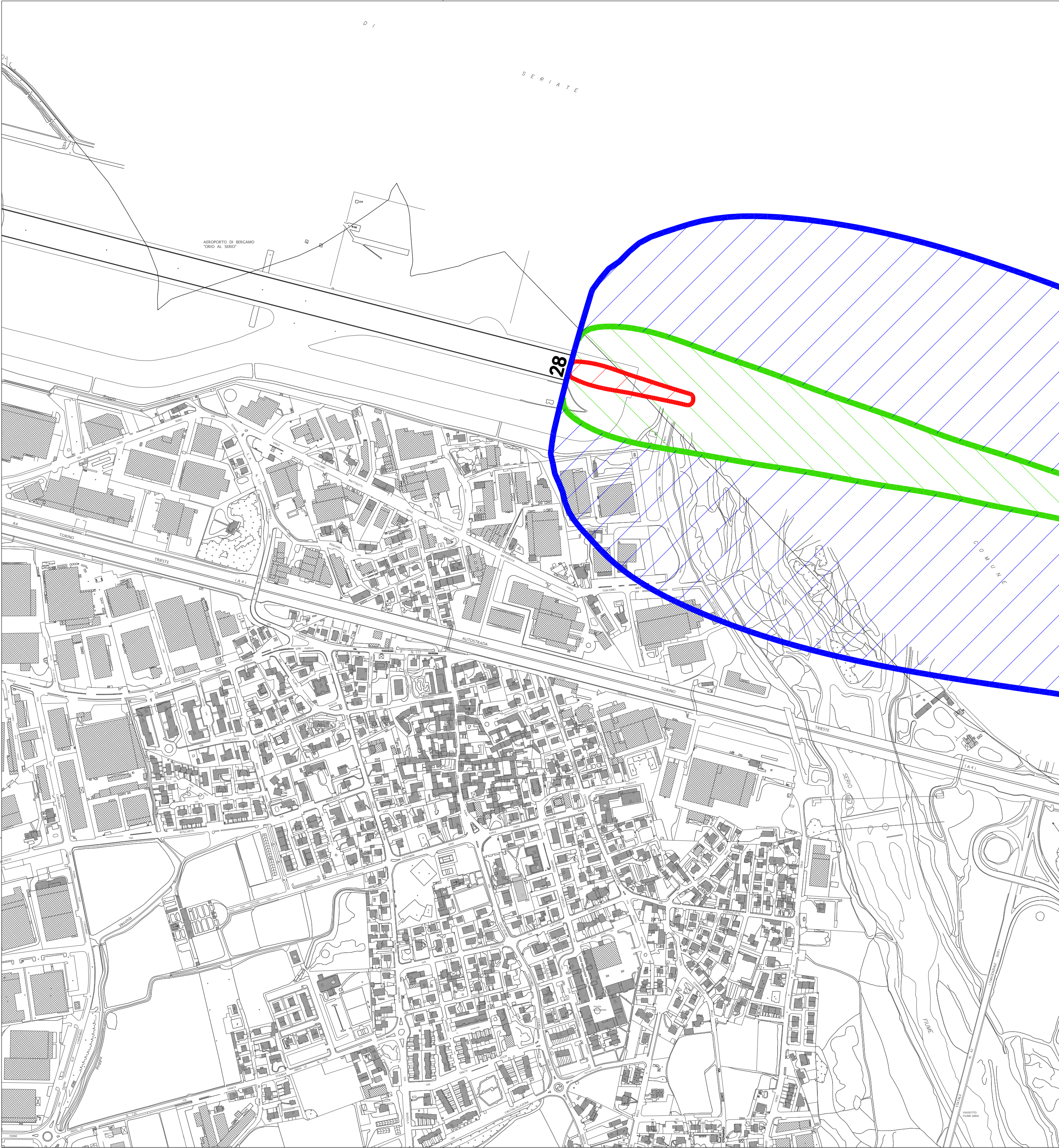
TAVOLA 3 INDIVIDUAZIONE DELLE AREE DEL THIRD PARTY RISK ASSESSMENT
