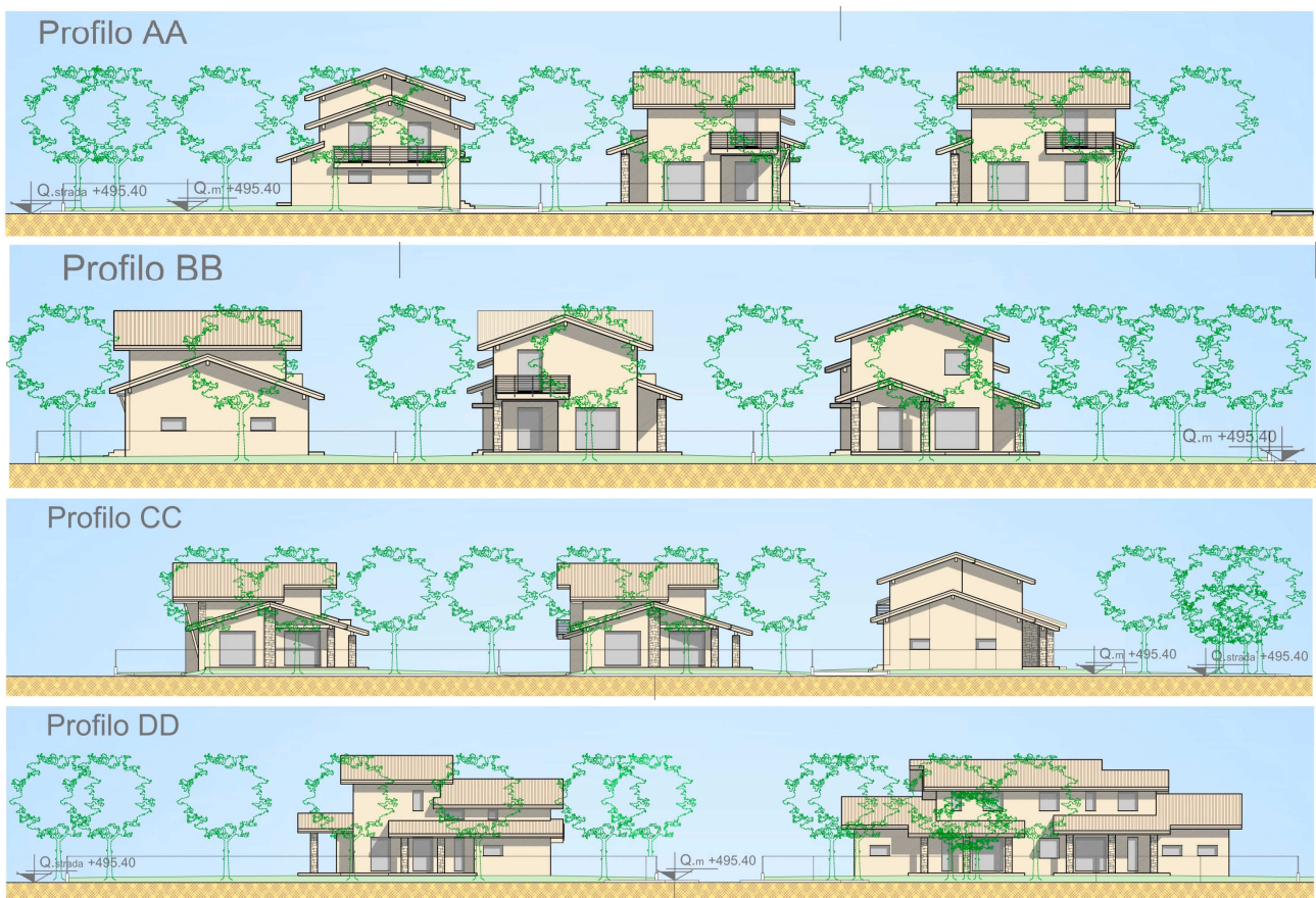
Stralcio Elaborato 2.0 P.E.C. – Profili di insieme (fuori scala)
