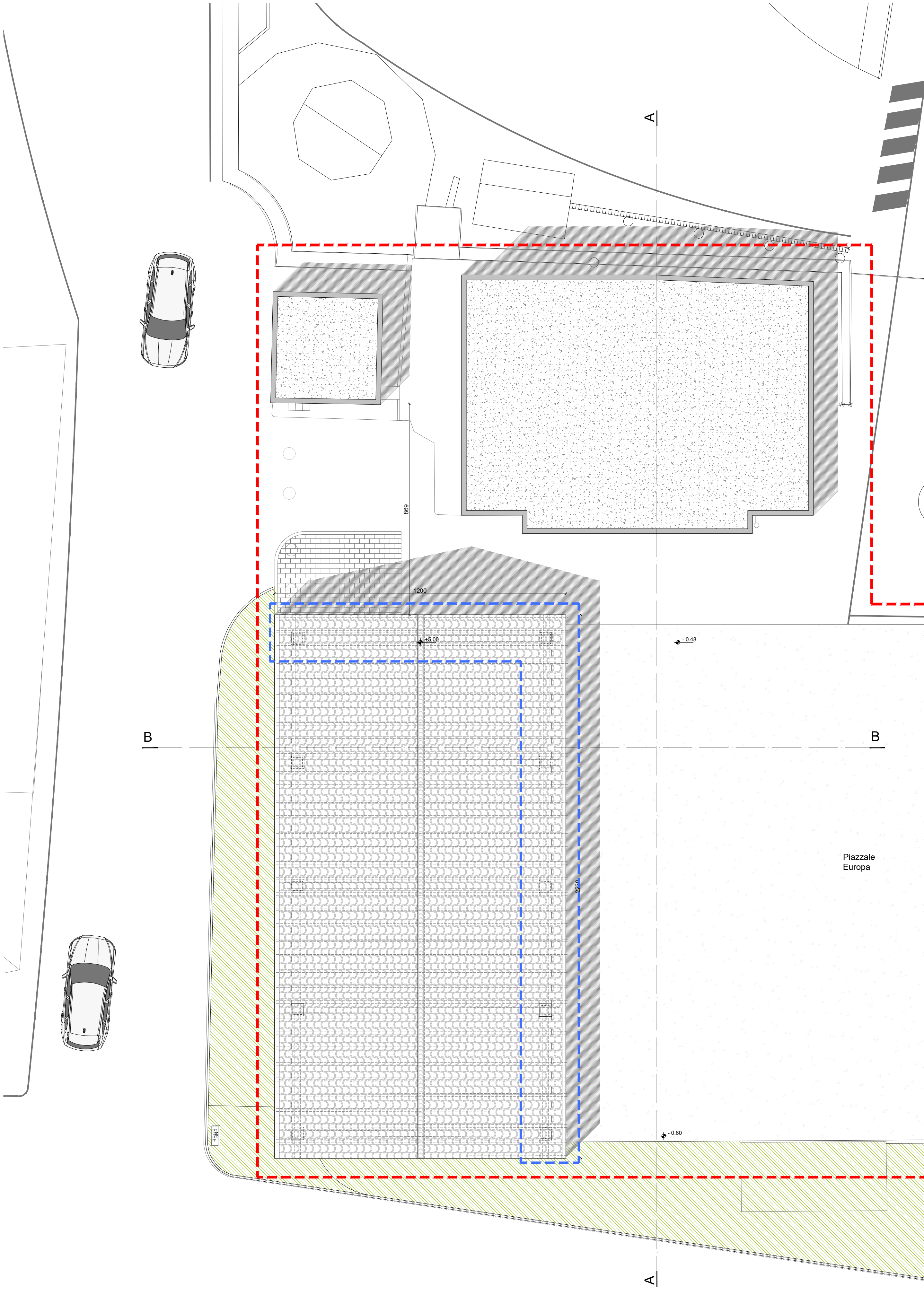
PIANTA COPERTURA
