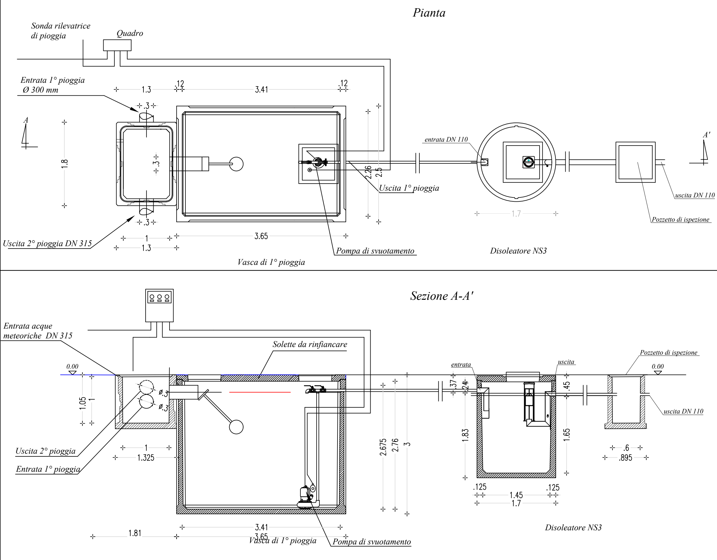
SCHEMA DEGLI SCARICHI DELLA GUARDIANIA 1:200
