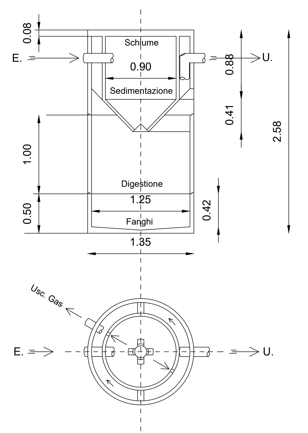
FOSSA IMHOFF 1:50
