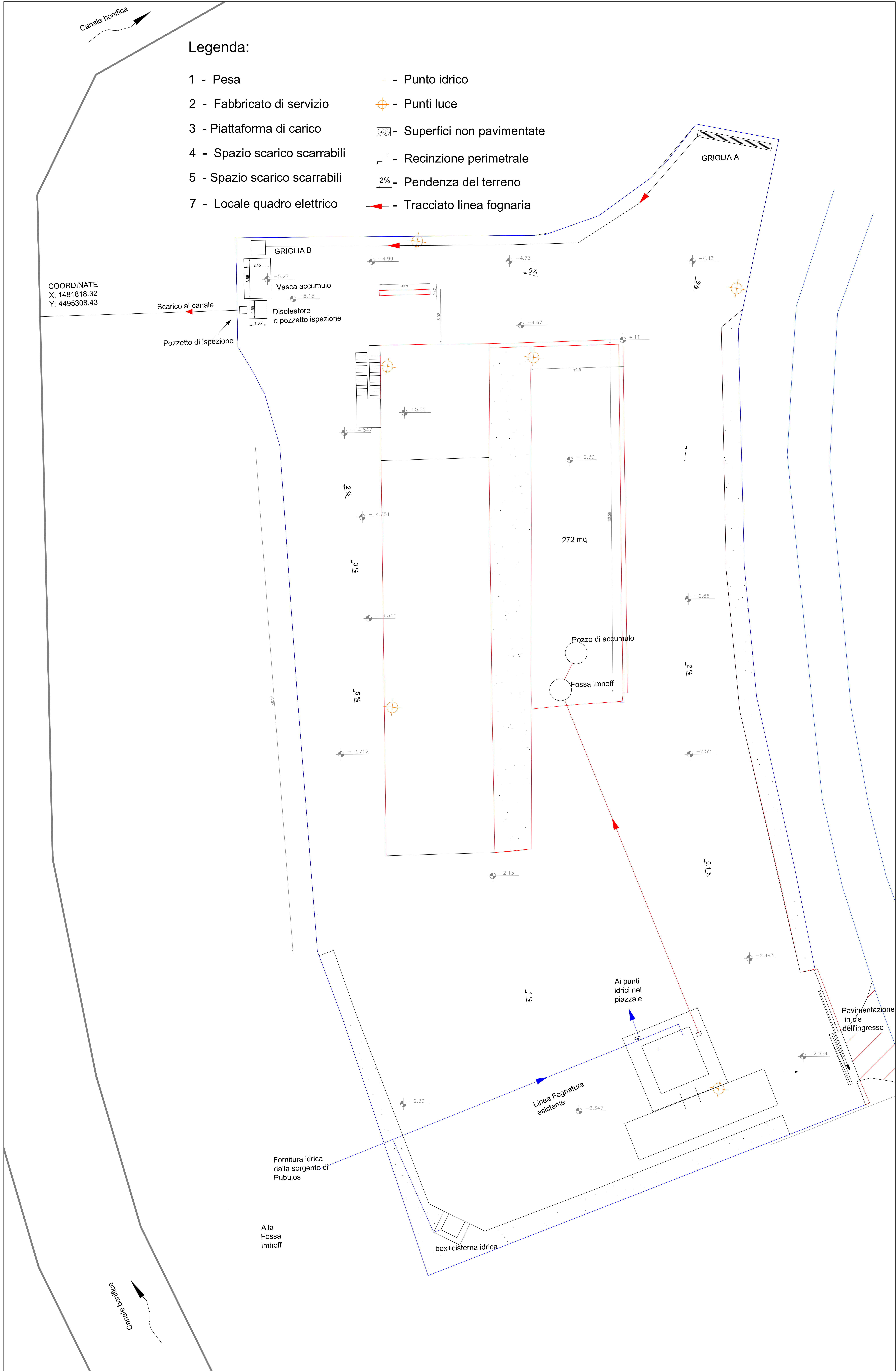
IMPIANTO PRIMA PIOGGIA 1:100
