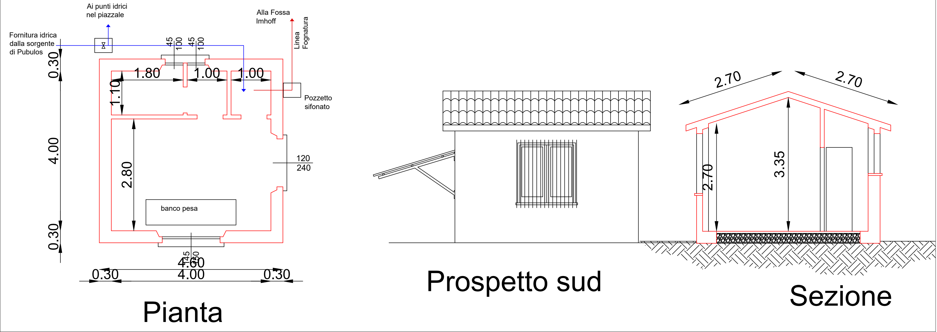
GUARDIANIA scala 1:100
