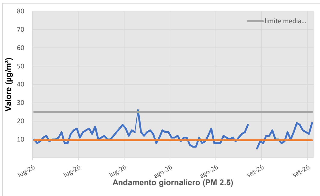
Figura 3: Concentrazioni giornaliere di PM2.5 (Valore limite 25 \mu\text{g}/\text{m}^3 su media annuale).
