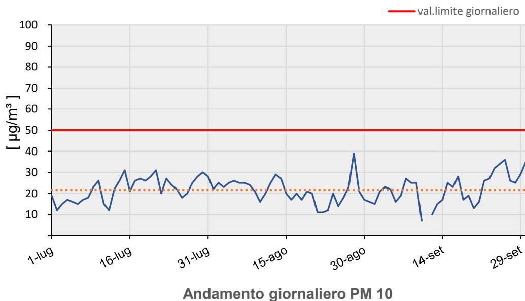
Figura 2: Concentrazioni giornaliere di PM10 (Valore soglia giornaliera: 50 \mu\text{g}/\text{m}^3 ).
