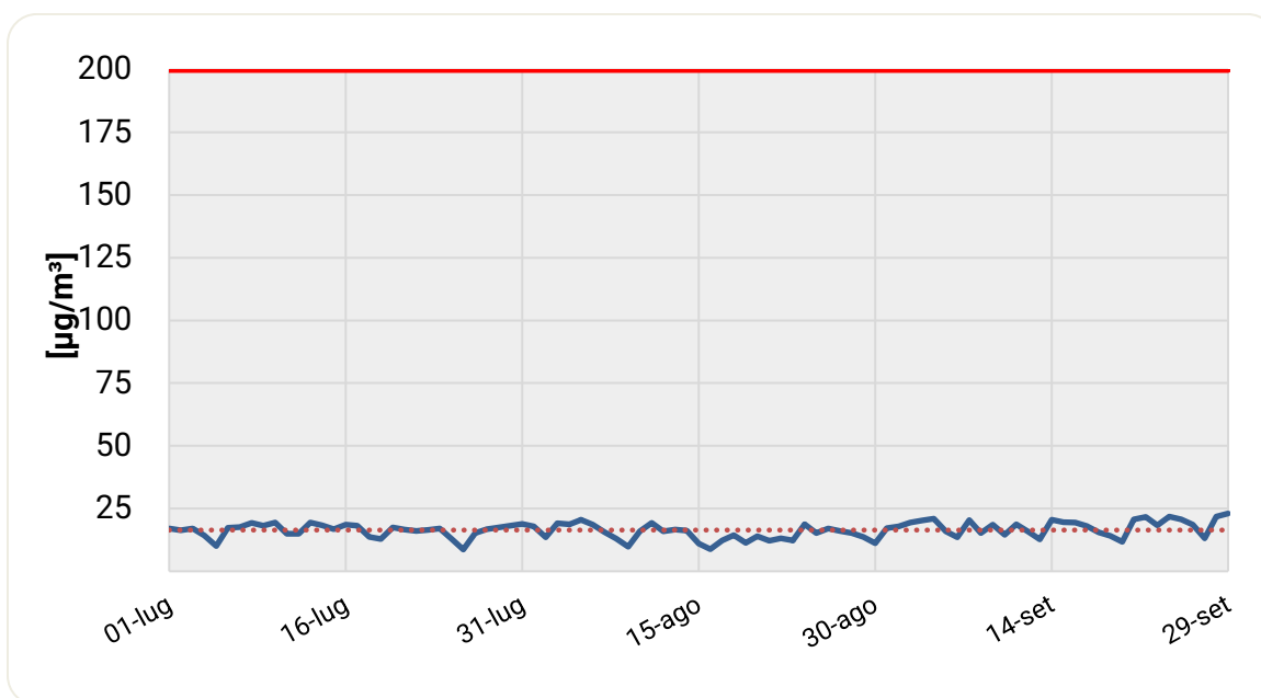
Figura 5: Concentrazioni medie giornaliere di NO 2 (Valore limite orario: 200 µg/m 3 ).
