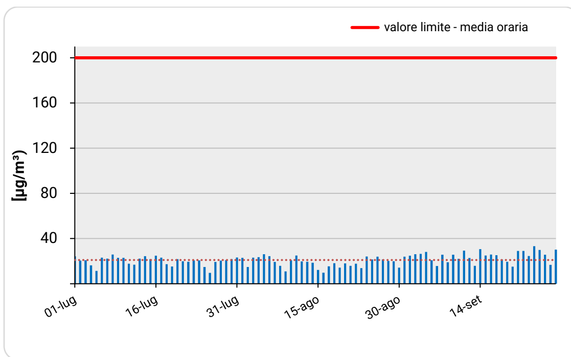
Figura 7: Concentrazioni medie giornaliere di NOx
