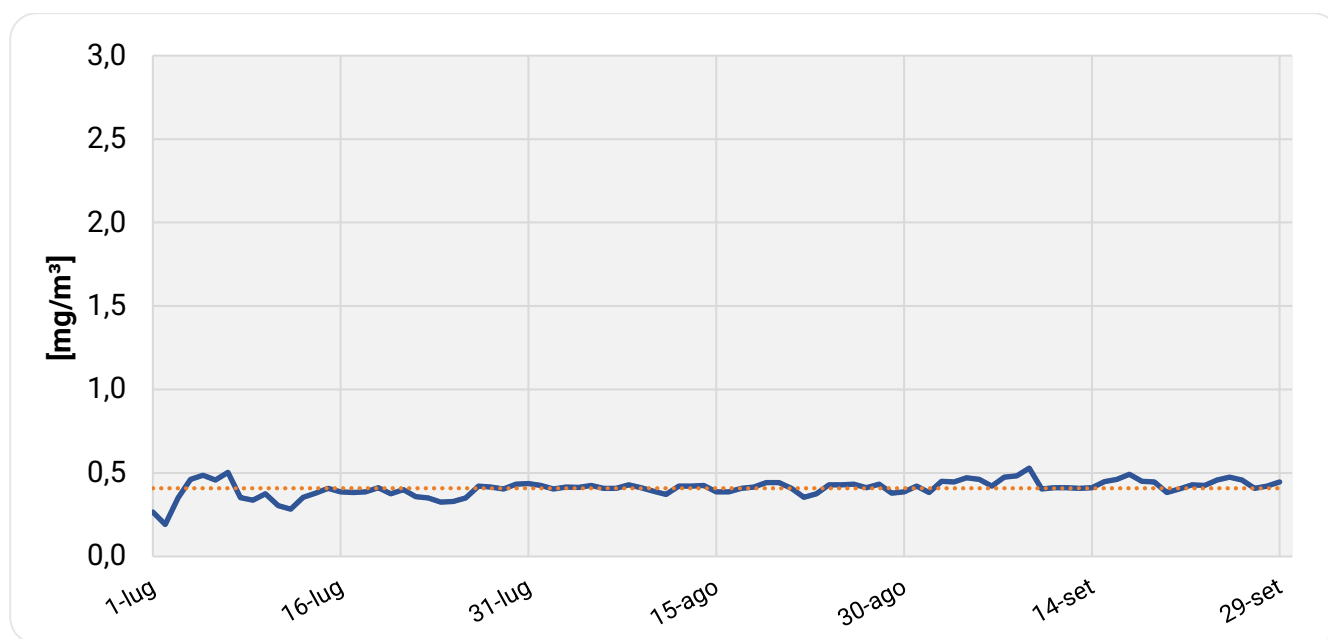
Figura 4: Concentrazioni medie giornaliere di CO (Valore limite 10 mg/m 3 ).
