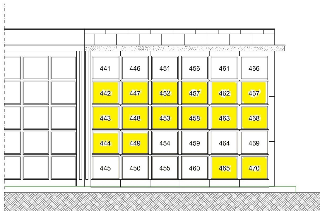
PROSPETTO FRONTALE
