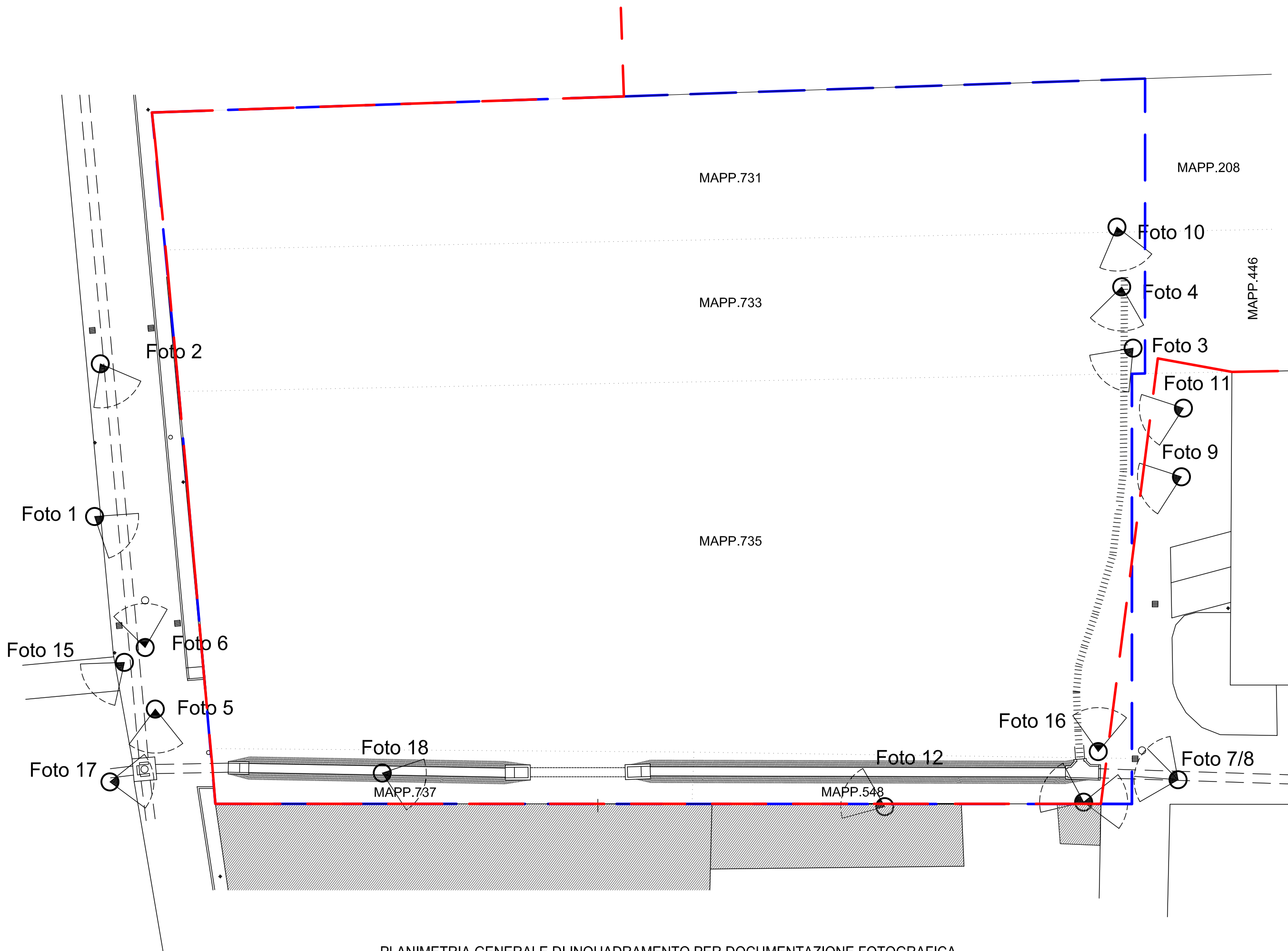
PLANIMETRIA GENERALE DI INQUADRAMENTO PER DOCUMENTAZIONE FOTOGRAFICA fuori scala
